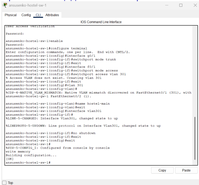
Рис.: Настройка интерфейсов коммутатора ansusenko-hostel-sw-1.
