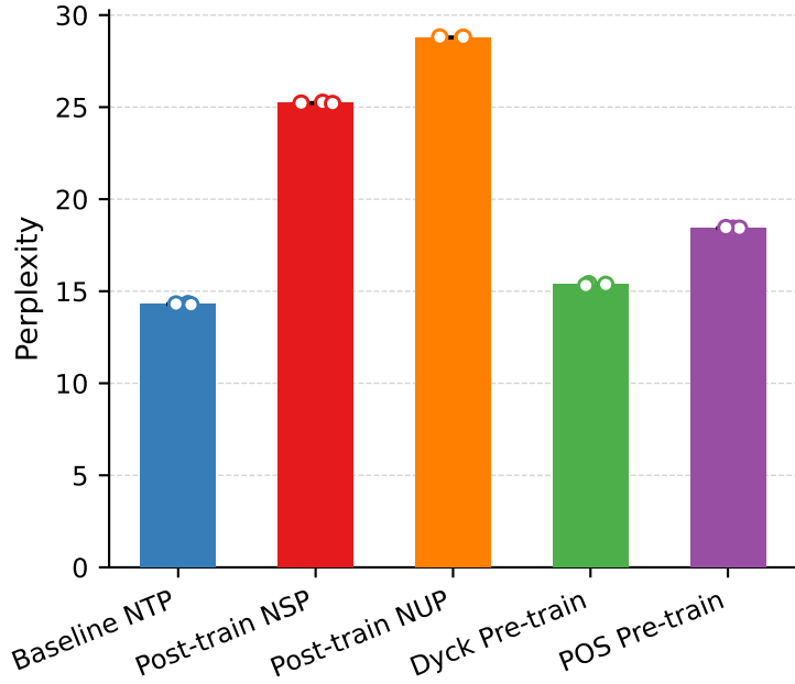
100M tokens
