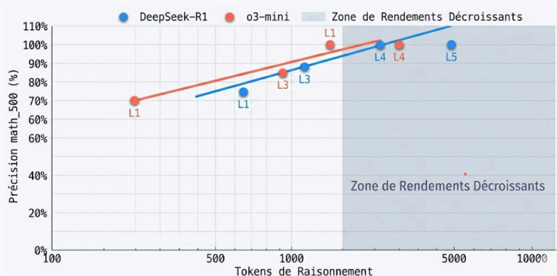
Corrélation entre précision et consommation de tokens de raisonnement. L’axe des ordonnées démontre la relation d’échelle non-linéaire.
