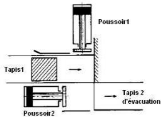
Figure 27. Système d'évacuation de pièces
