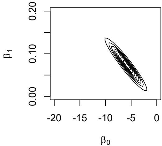
Joint Posterior
