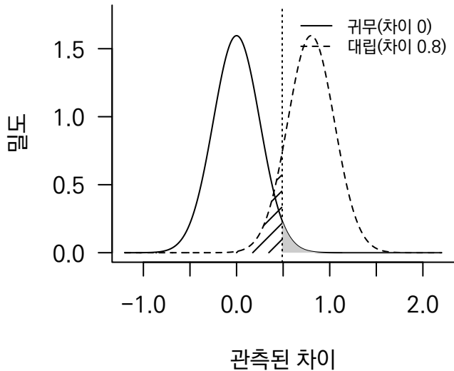
(a) 두 분포의 겹침
