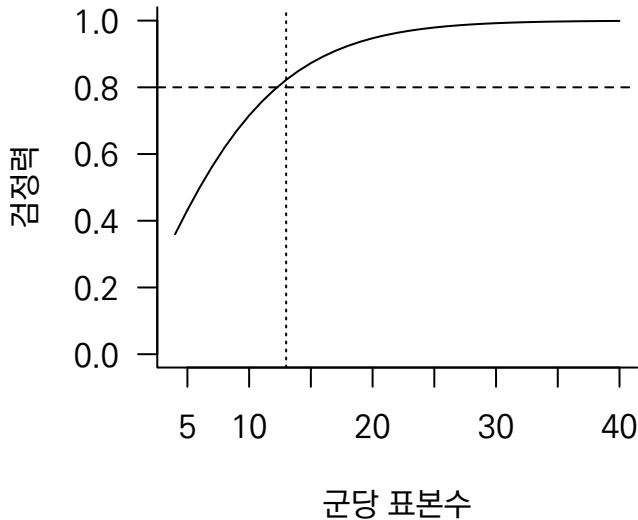
(b) 검정력 곡선
