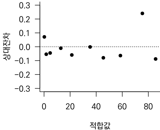
(b) WLS
