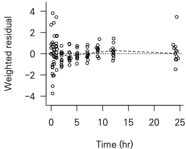
(a) WRES (eta = 0 전개)
