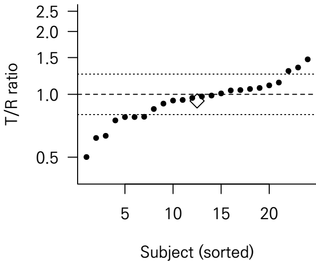
AUClast
