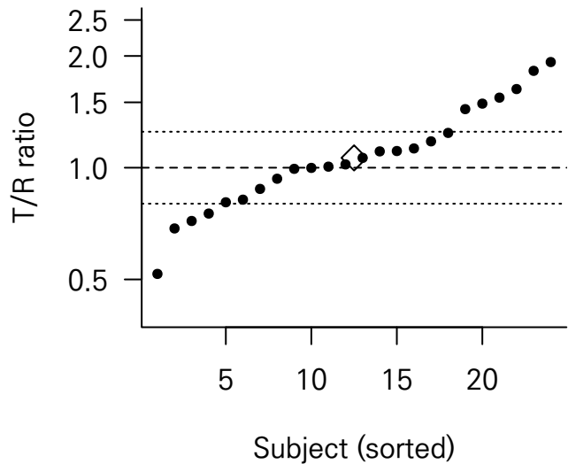
Cmax
