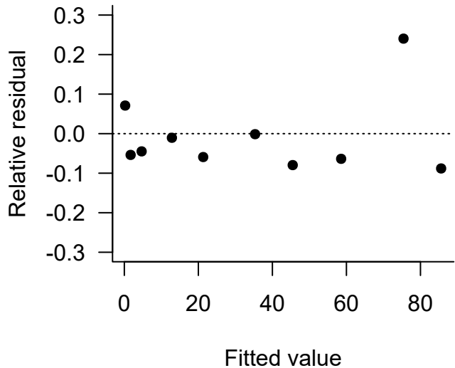
(b) WLS
