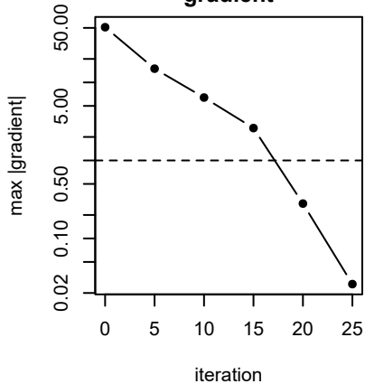
gradient
