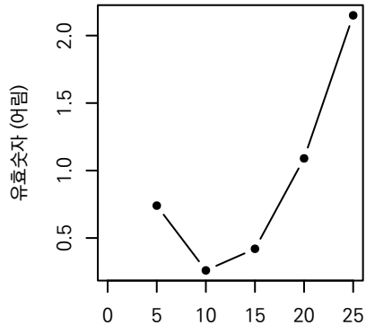
유효숫자
