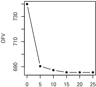
목적함수
