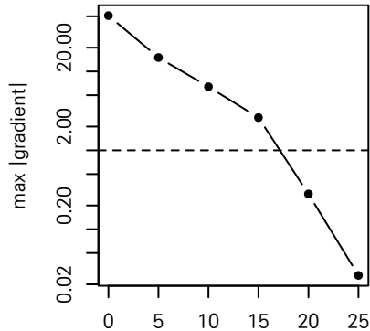
gradient
