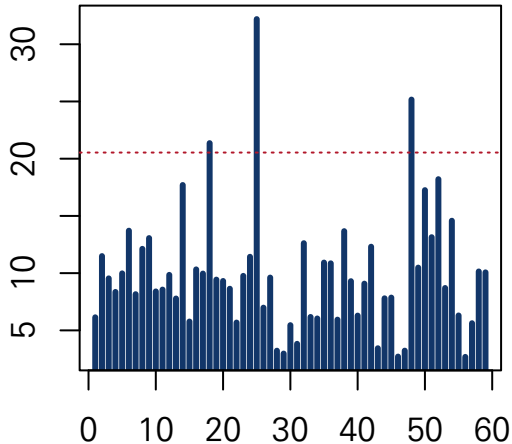
개인 목적함수값
