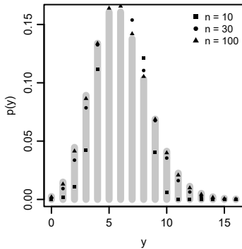
Bin(n, 6/n) -&gt; Pois(6)
