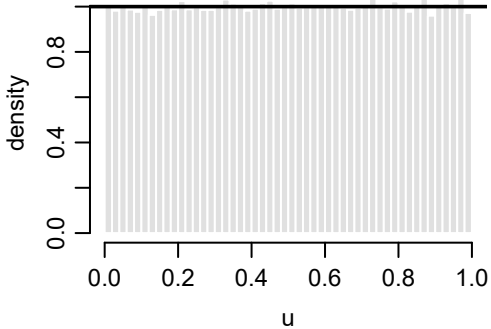
runifLC(1e5)
