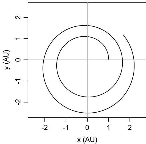
Euler
