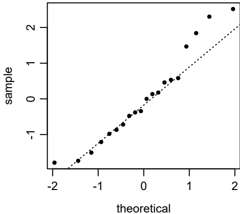
normal Q-Q
