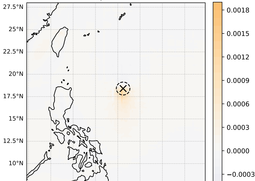
850 hPa vorticity ( \text{s}^{-1} , max = 1.84\text{e-}03 )
