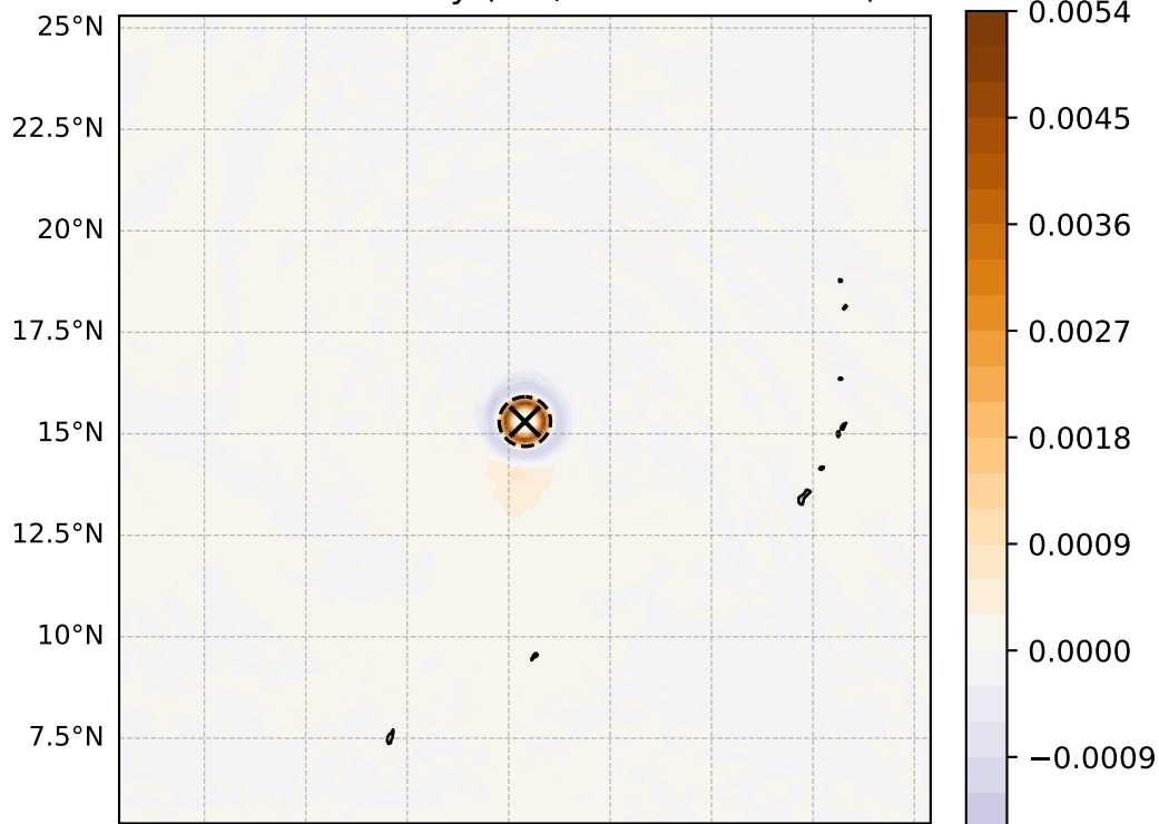
850 hPa vorticity ( \text{s}^{-1} , max = 5.12\text{e-}03 )
