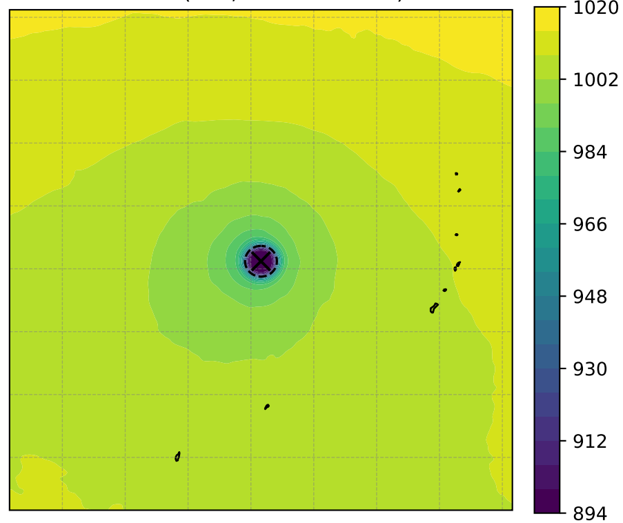
MSLP (hPa, min = 897.00)
