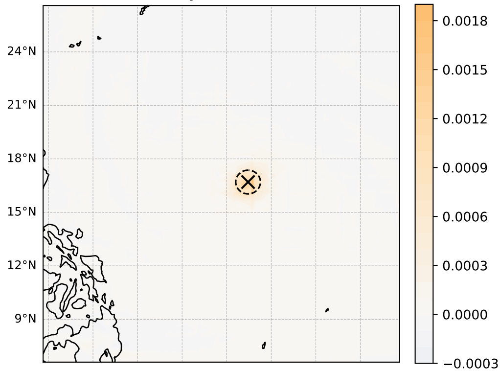
850 hPa vorticity ( \text{s}^{-1} , max = 1.84\text{e-}03 )
