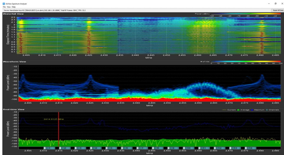
Figura 5: Captura ilustrativa del analizador de espectro airView . b4
