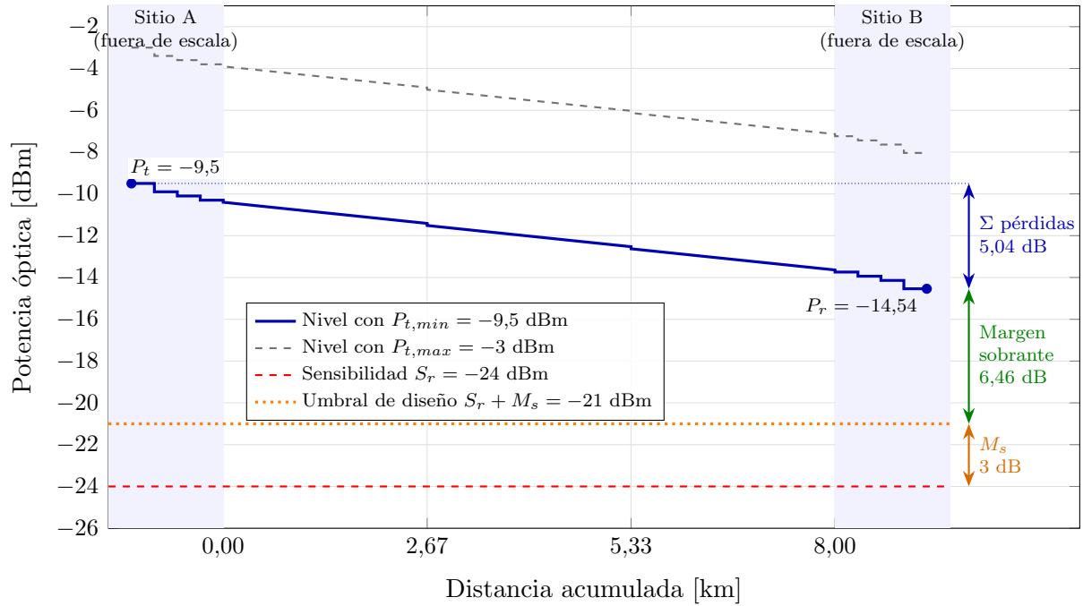
Figura 4: Presupuesto óptico del enlace: nivel de potencia a lo largo del trayecto (sentido A \rightarrow B).
