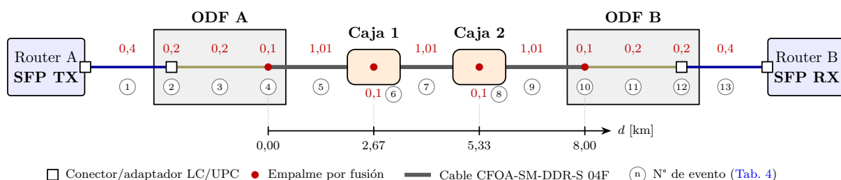
Figura 3: Esquema del enlace (una fibra, sentido A \rightarrow B) con la pérdida de cada evento en [dB] (en rojo) y la distancia acumulada. Los elementos internos de cada sitio se representan fuera de escala.
