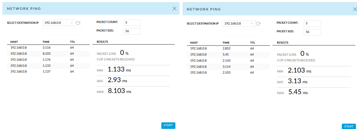
(a) Ping con las antenas alineadas
