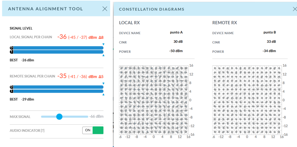
(a) Antenas alineadas
