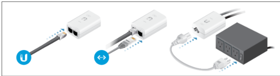
Figura 8: Adaptador PoE.
