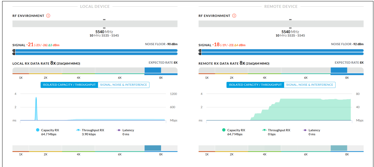
Figura 18: Panel principal del enlace en el pasillo
