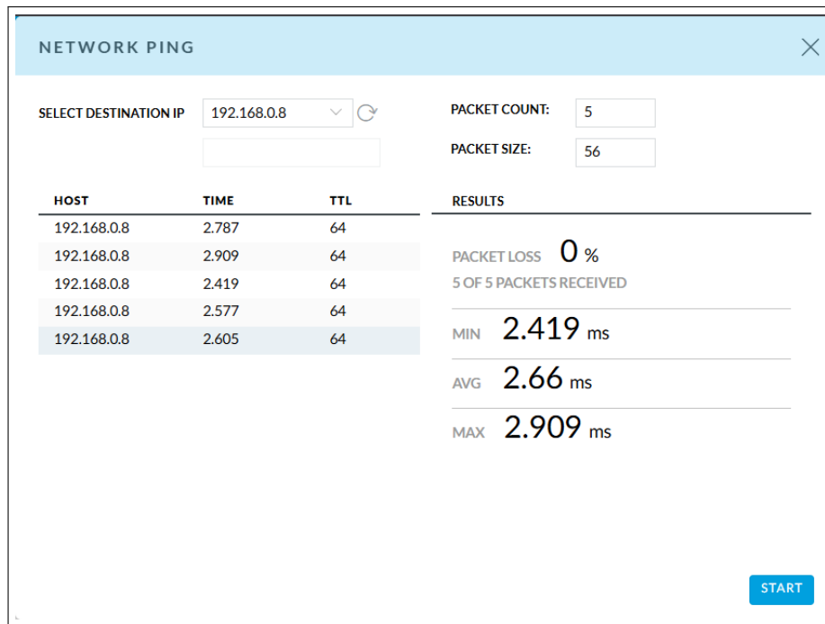
Figura 26: Prueba de ping con canal de 10 MHz (Alineado)
