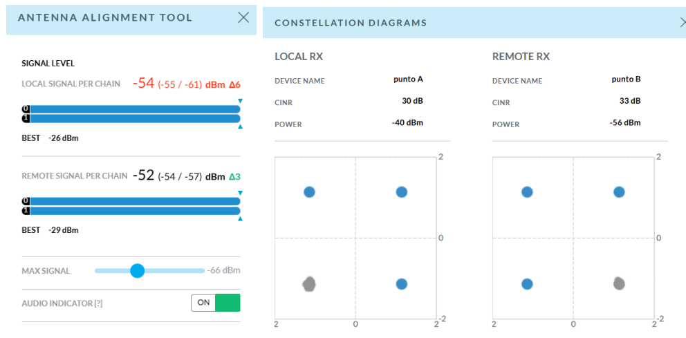
(a) Antenas desalineadas
