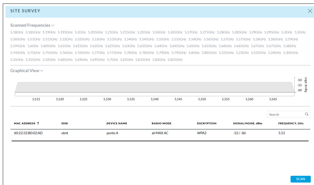
Figura 15: Captura del resultado de Site Survey
