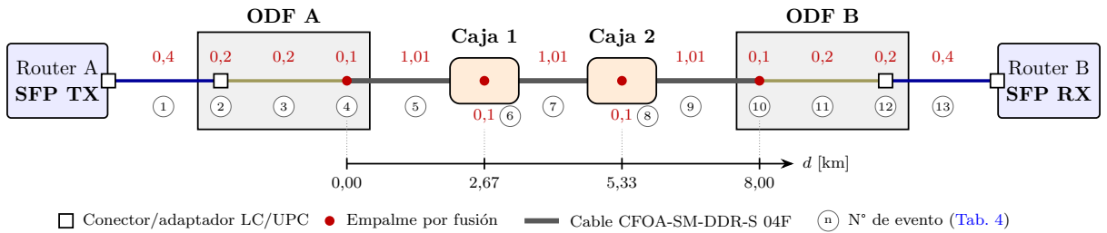
Figura 3: Esquema del enlace (una fibra, sentido A \rightarrow B) con la pérdida de cada evento en dB (en rojo) y la distancia acumulada. Los elementos internos de cada sitio se representan fuera de escala.
