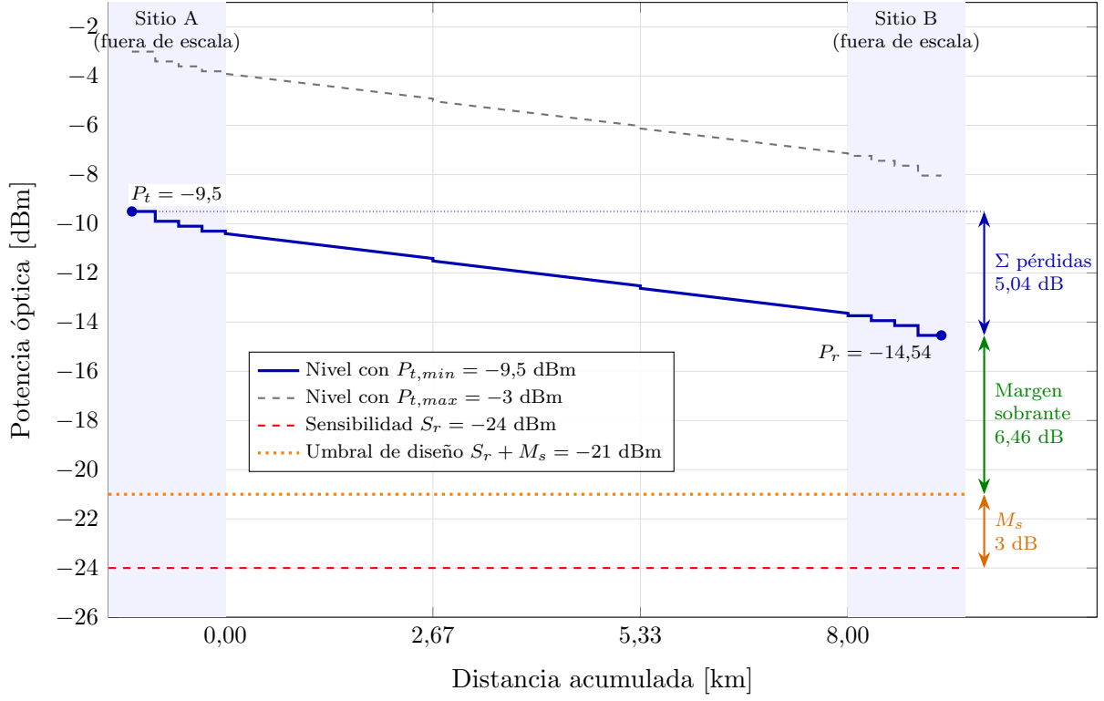
Figura 4: Presupuesto óptico del enlace: nivel de potencia a lo largo del trayecto (sentido A \rightarrow B ).
