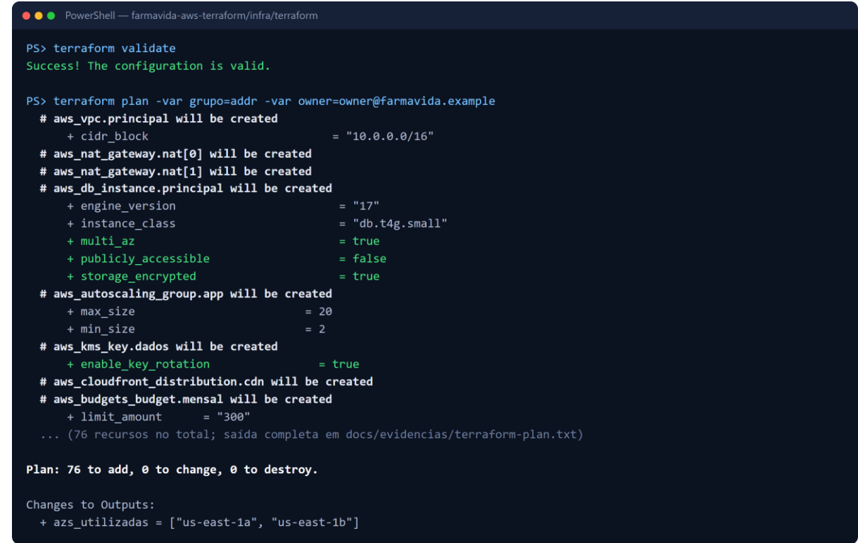
Figura 2 — terraform validate e trechos do terraform plan (saída completa em docs/evidencias/terraform-plan.txt, com o ID da conta mascarado).
