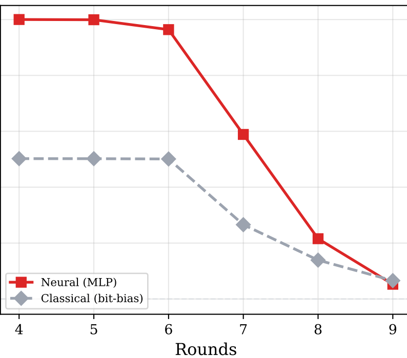
SIMON32/64 (Feistel)
