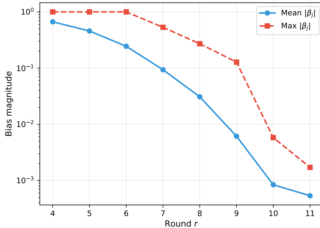
SIMON32/64 (Feistel)
