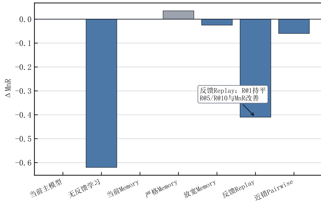
(b) 平均排名 MnR 变化 (越低越好)
