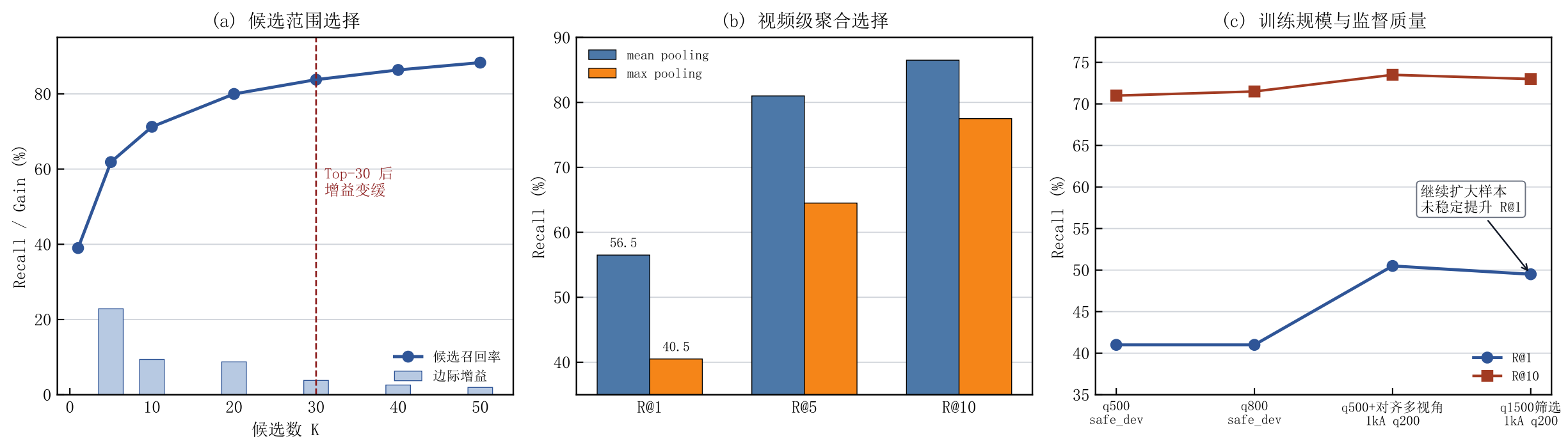
图3-4 关键实验设置选择的消融分析
