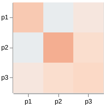
ZImageTurbo → LLaMA32Vision
