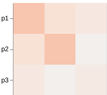
GLMImage → LLaMA32Vision
