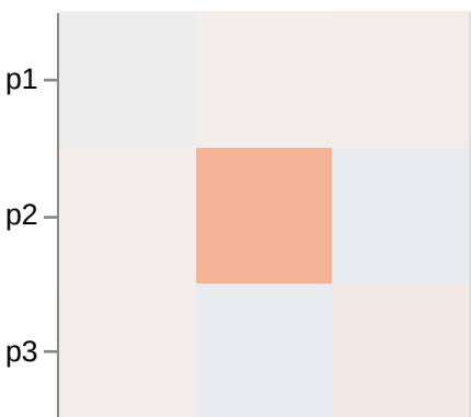
SD35Medium → Moondream
