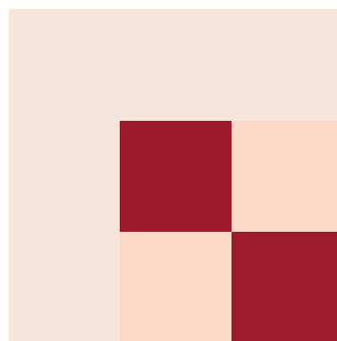
ZImageTurbo → Gemma3n
