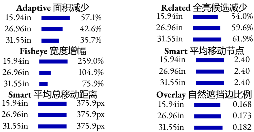
图 5.7: 显示优化功能随屏幕尺寸配置变化的效果
