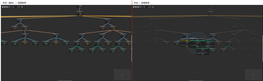
图 5.5: 鱼眼聚焦关闭与开启：概览中恢复目标尺寸并淡化远处节点
