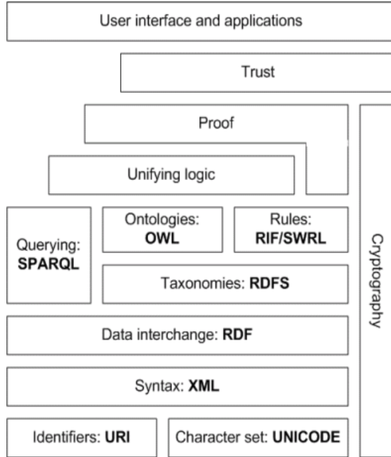
الشكل (1) طبقات الويب الدلالي [23]
