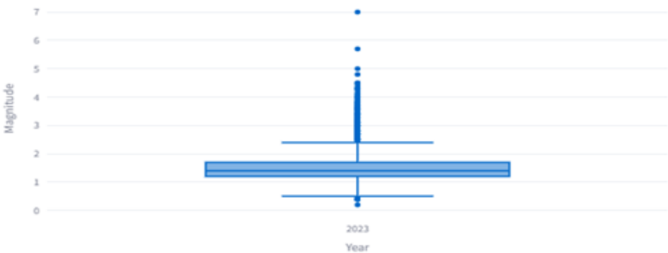
Boxplot de la magnitude par rapport à l'année
