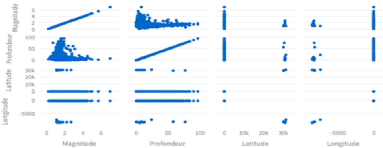
Pairplot des variables numériques
