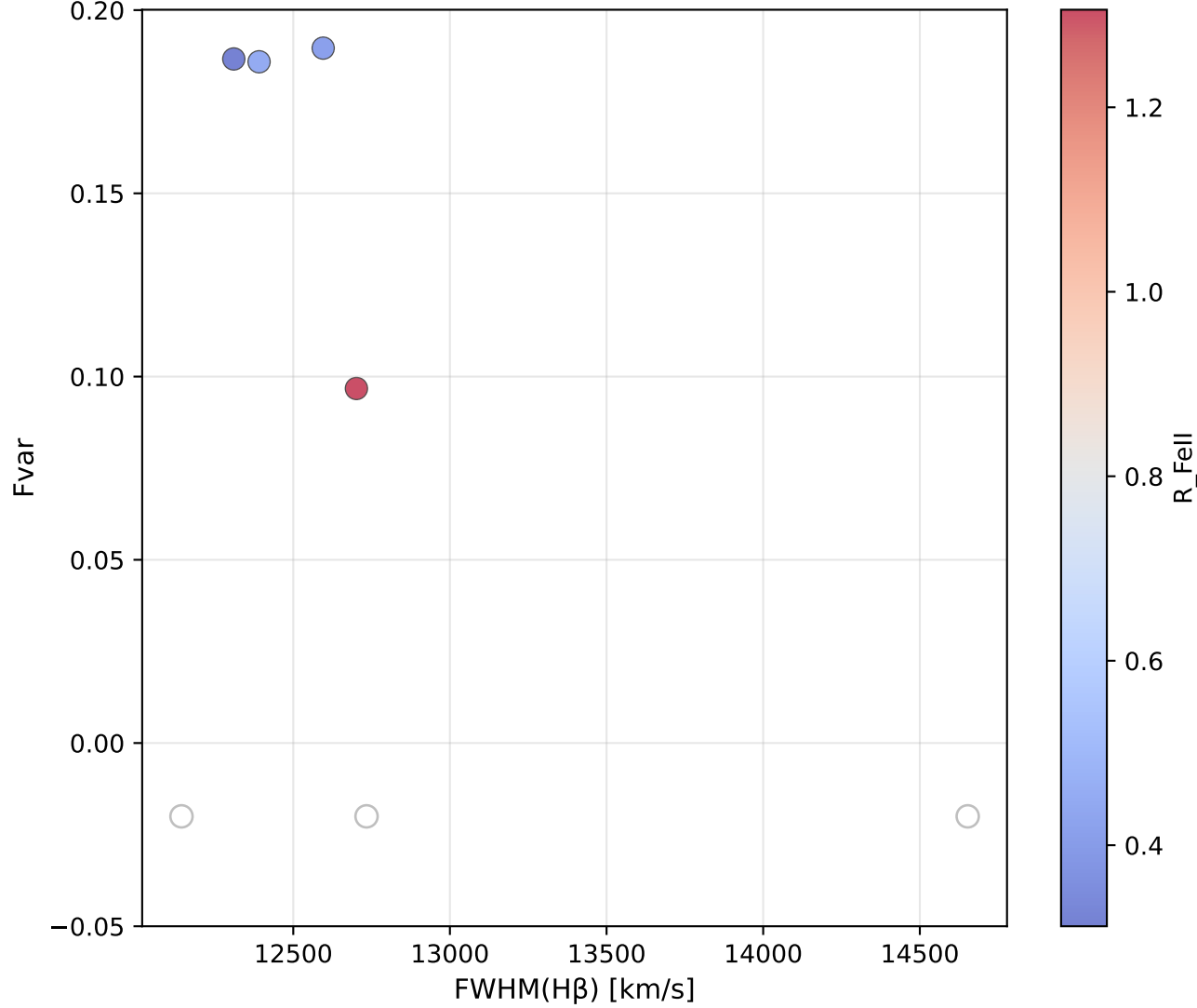
ALERCE fid=2 (N=4 det, 3 non-det)
