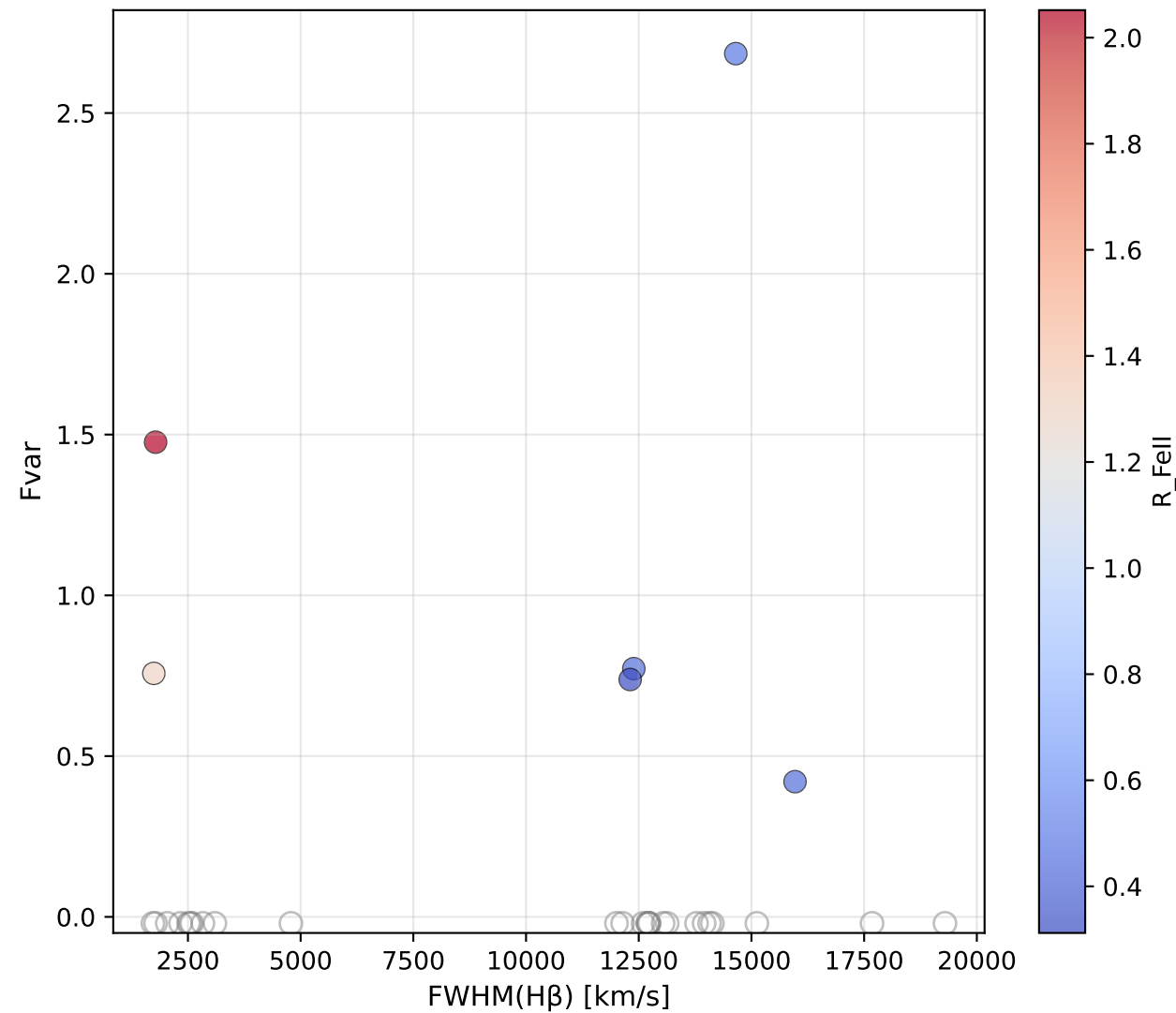
ALERCE fid=2 (N=4 det, 3 non-det)
