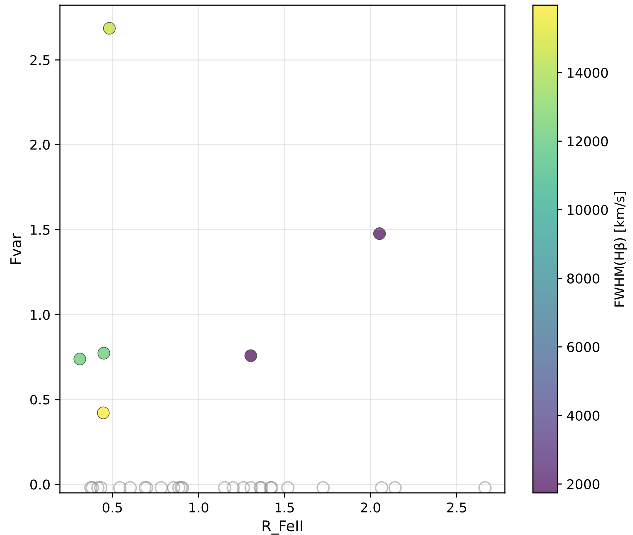
ALERCE fid=2 (N=4 det)
