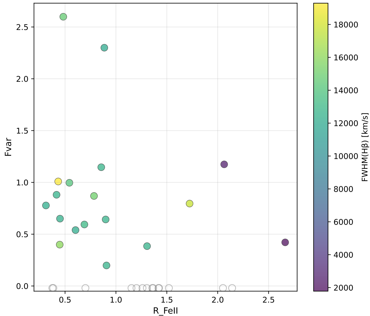
ALERCE fid=1 (N=5 det)
