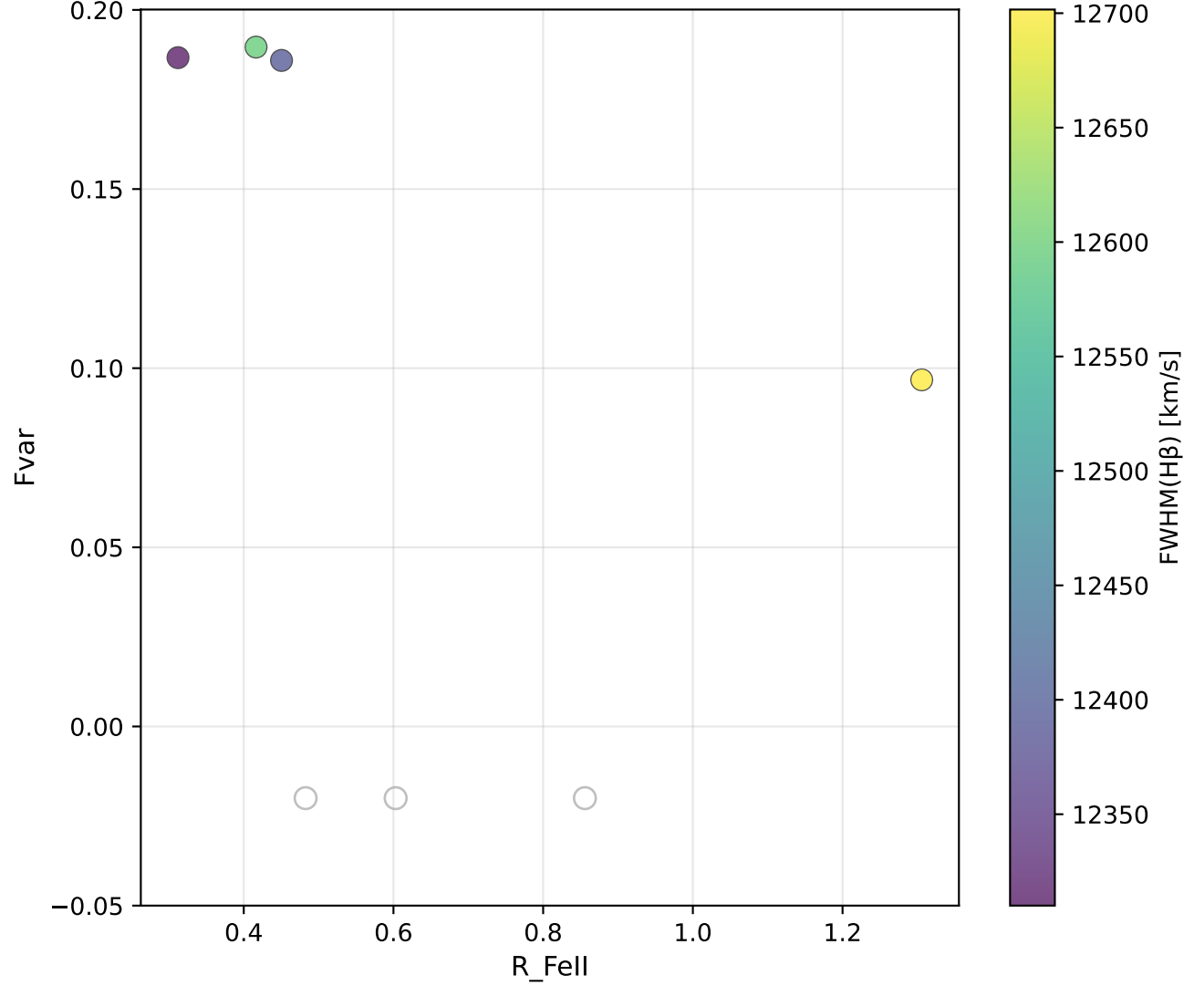
ALERCE fid=2 (N=4 det)
