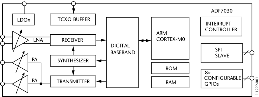
图 1.2 图 1.2 ADF7030 框图 [3]
