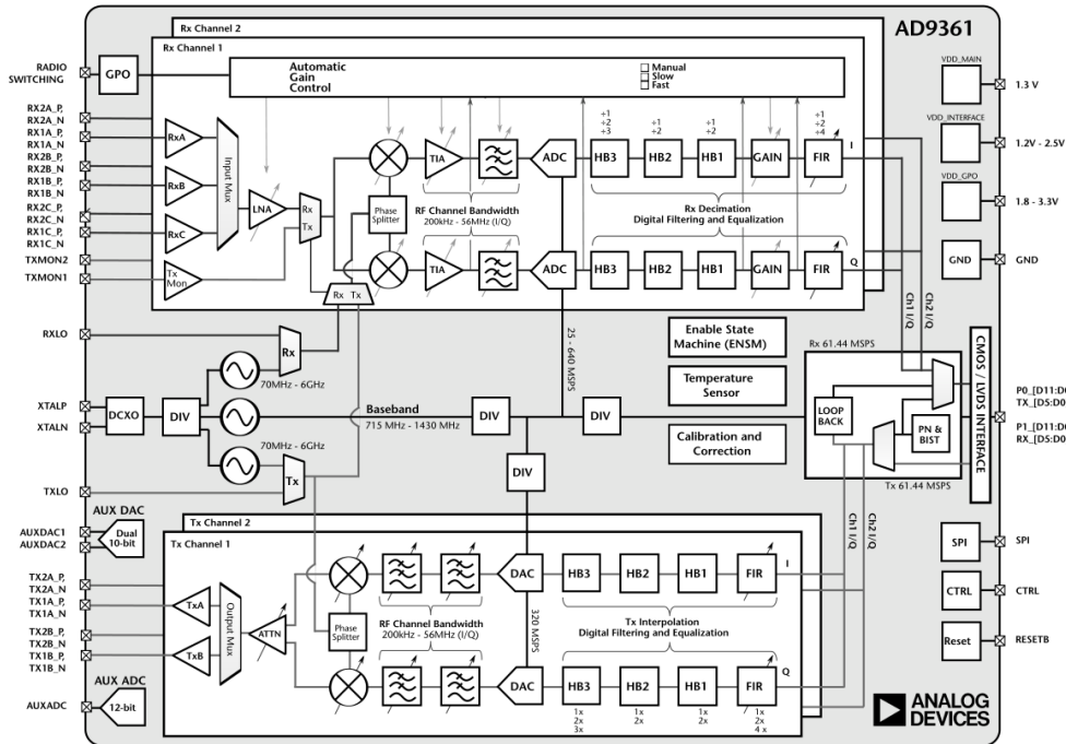
图 1.8 图 1.8 Pluto SDR 所用的集成 ZIF 架构
