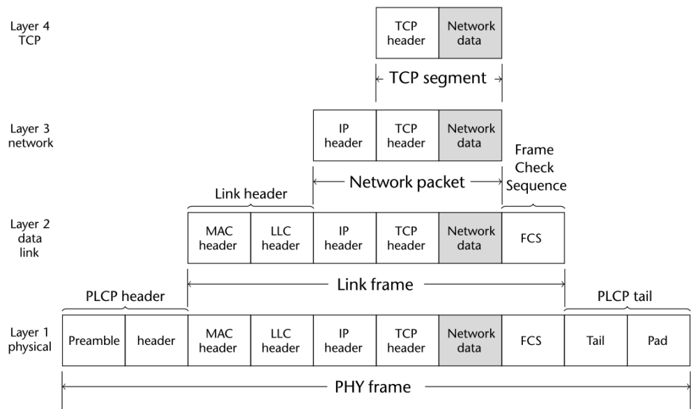
图 1.5 图 1.5 分组结构对 SDR 的影响，PLCP = 物理层收敛协议
