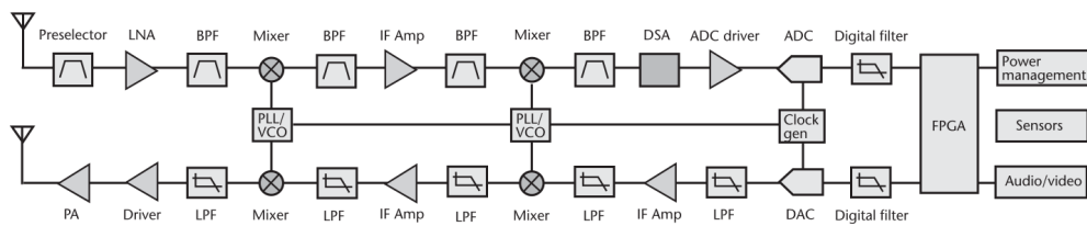
图 1.6 图 1.6 多级超外差接收与发射信号链 [4]
