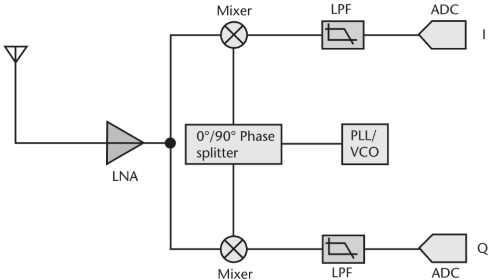
图 1.7 零中频架构 [4]
