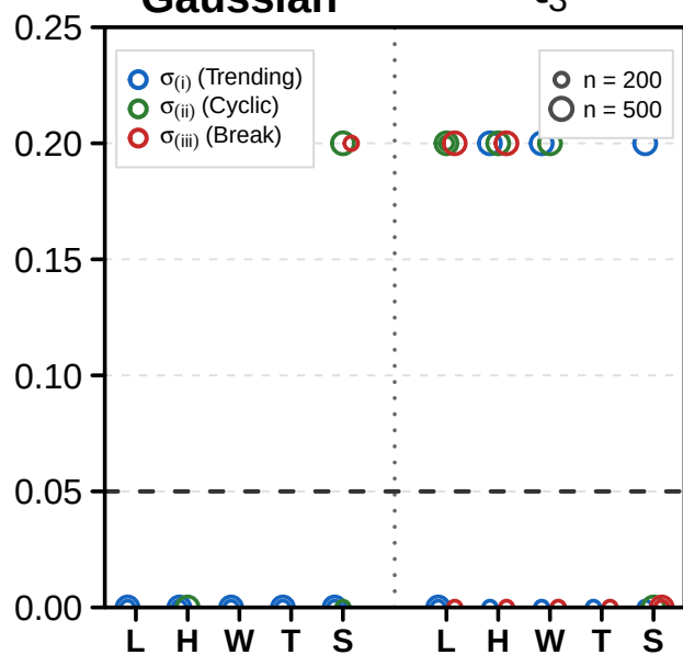
H 0 : No Shift (Size)
