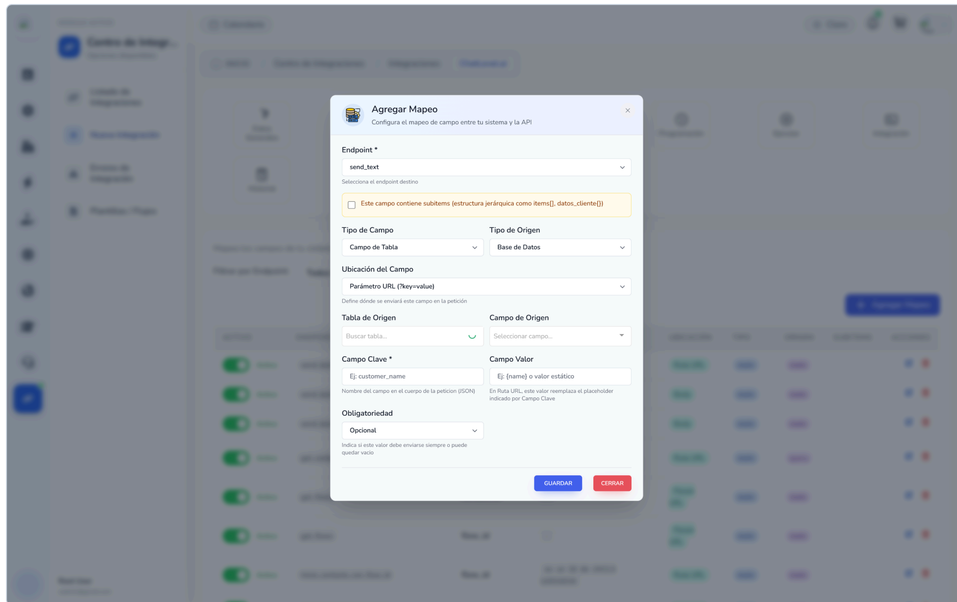
Figura 12. Modal «Agregar Mapeo»: endpoint, tipo de campo, tipo de origen, tabla y campo de origen, ubicación del campo, valor por defecto, obligatoriedad y la sección de subitems para estructuras Object o Array .
