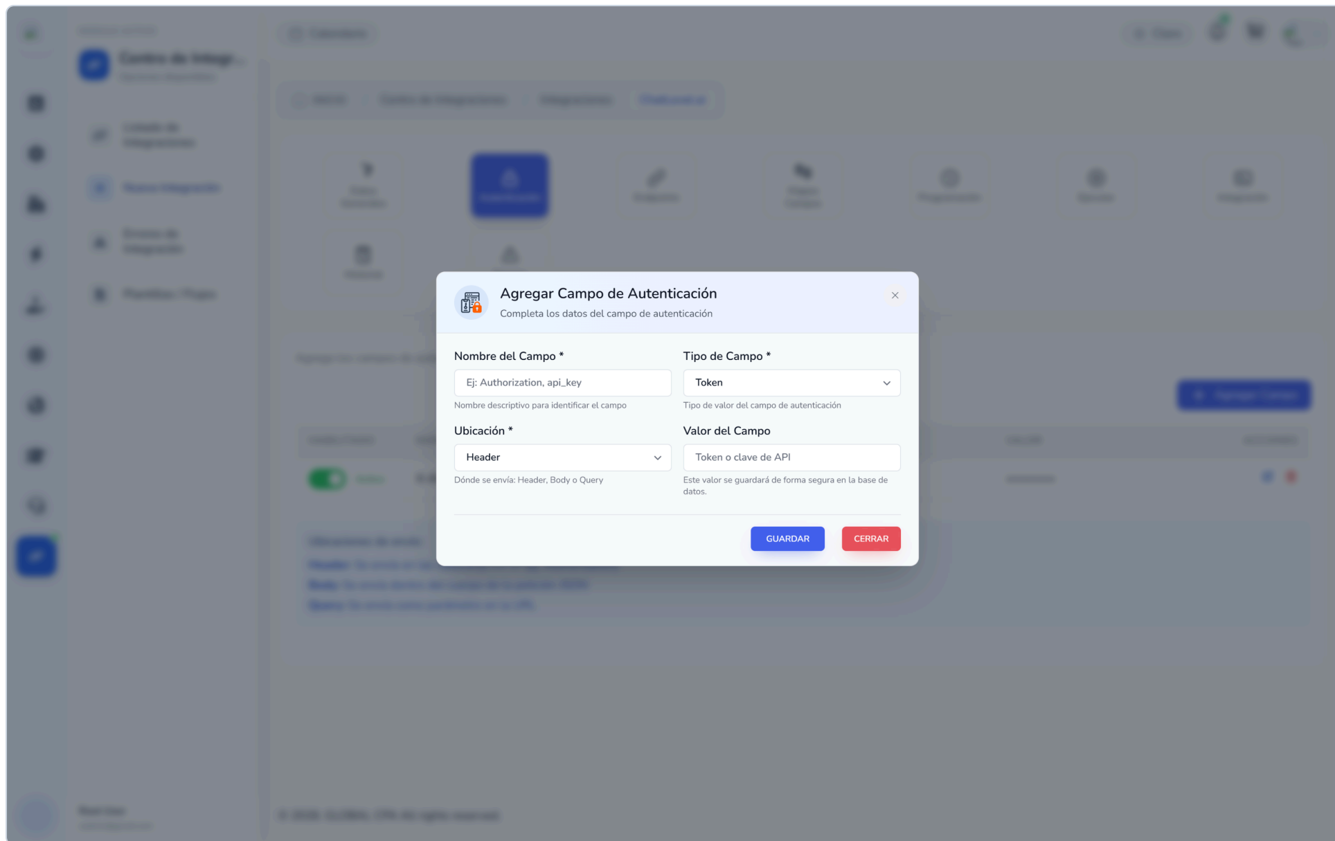
Figura 8. Modal «Agregar Campo de Autenticación». Al elegir el tipo Basic Auth aparecen los campos Usuario y Contraseña, y el sistema arma la cabecera Basic automáticamente.
