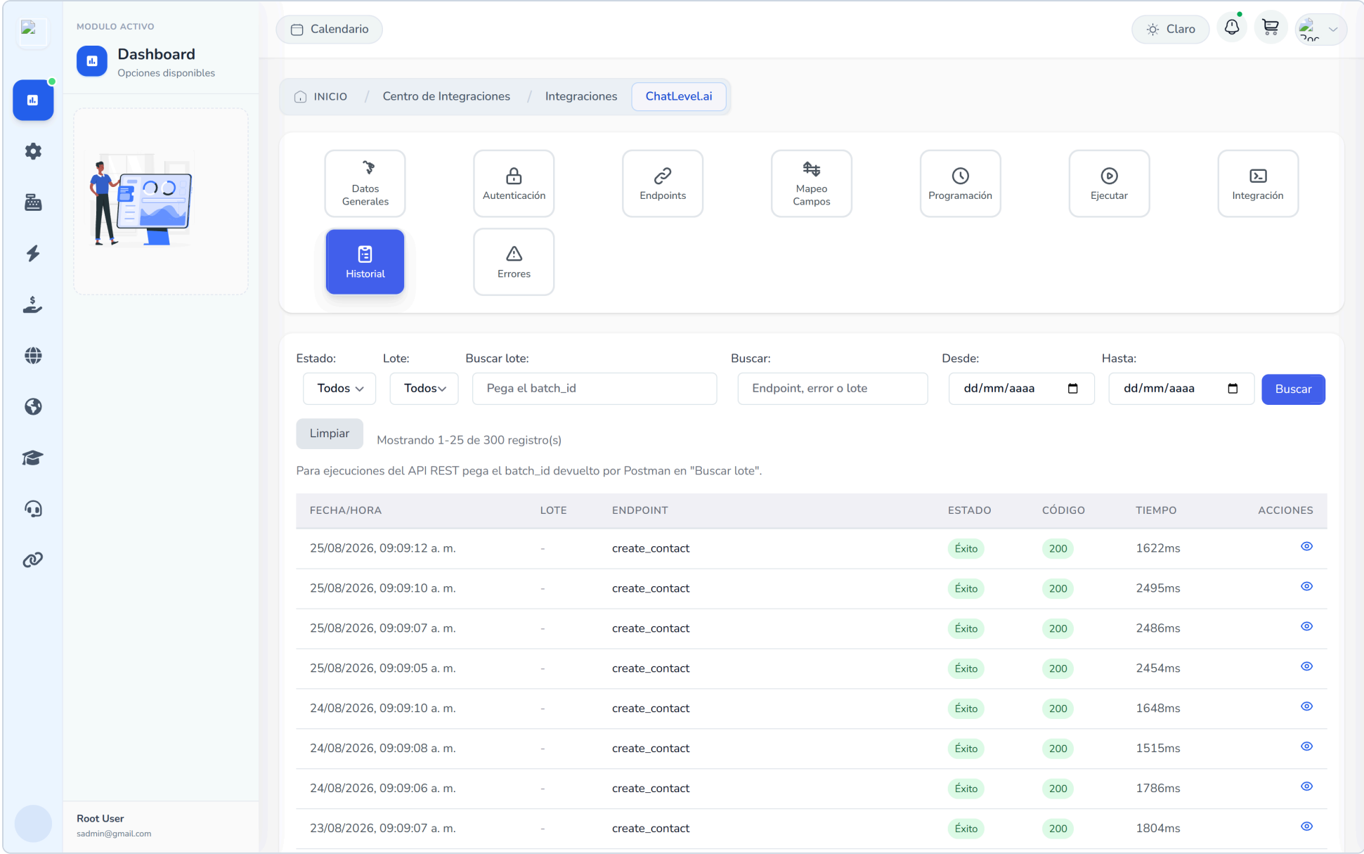
Figura 17. Historial real de ChatLevel.ai: fecha y hora, lote, endpoint, estado, código HTTP y tiempo de ejecución (milisegundos) de cada llamada.
