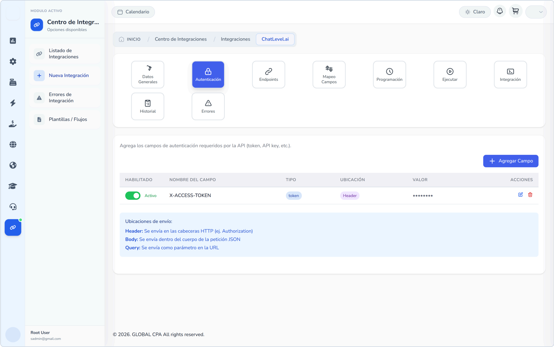
Figura 7. Pestaña Autenticación con la credencial real de ChatLevel.ai: cabecera X-ACCESS-TOKEN de tipo token, habilitada. Se puede editar, activar/desactivar o eliminar cada campo.
