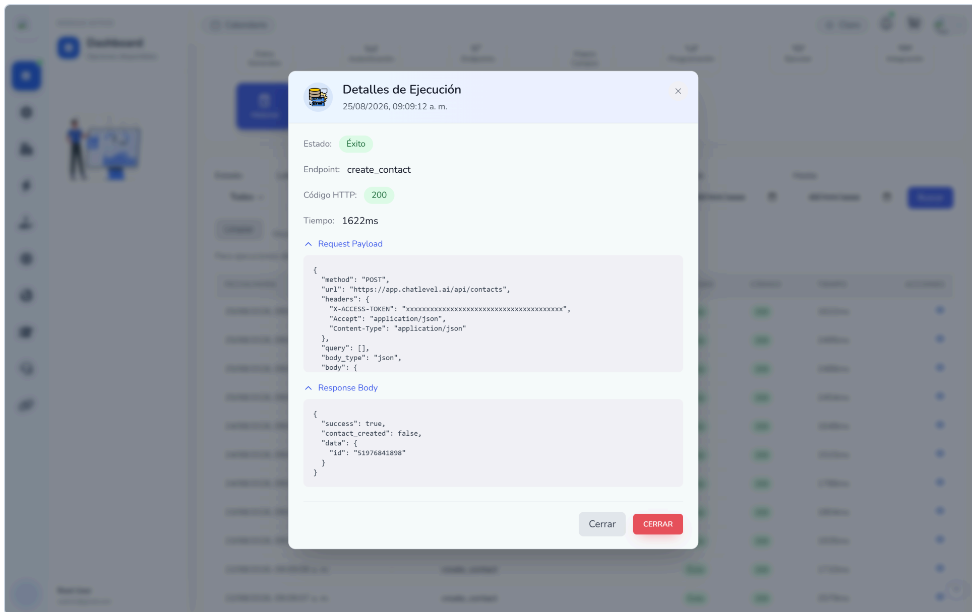
Figura 18. Detalle de una ejecución real: estado, endpoint, código HTTP, tiempo, y los bloques desplegable Request Payload y Response Body . Se aprecia el enmascarado del token de acceso (todo x ) mientras el resto de la petición y la respuesta se guardan completos.
