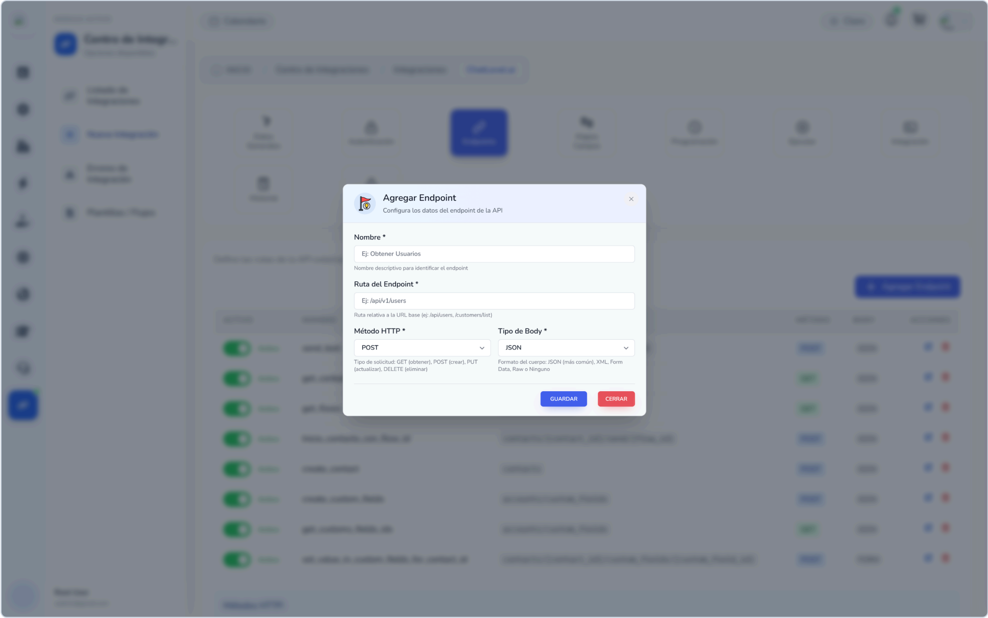
Figura 10. Modal «Agregar Endpoint». El método arranca en POST y el tipo de cuerpo en JSON. La ruta acepta marcadores con llaves cuando el mapeo de campos usa la ubicación «Ruta URL».
