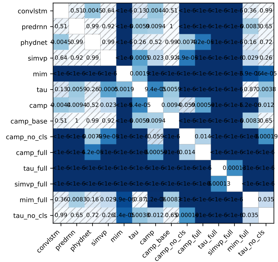
Paired t-test p-values (metric = MAE)
