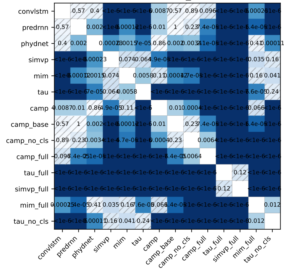
Paired t-test p-values (metric = POI_MAE)
