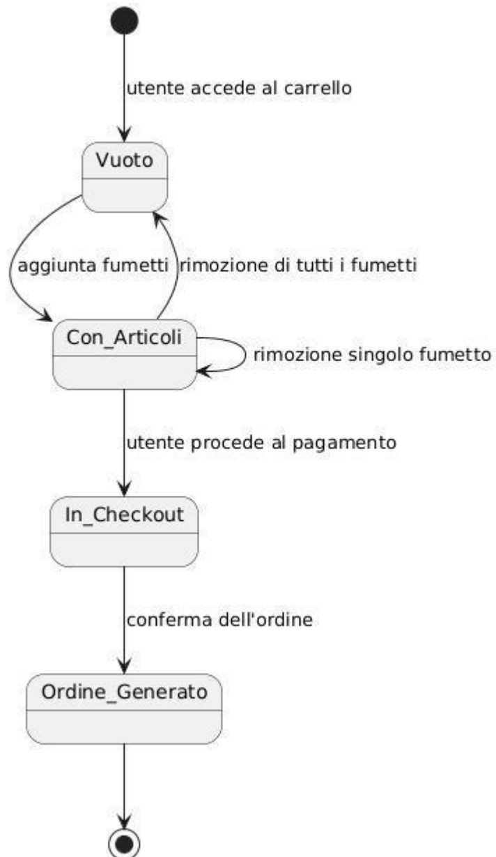
Diagramma di Stato - Carrello (FumettoVerse)
