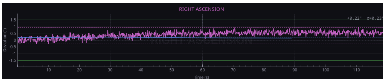
FIGURE 3.1 – Le graphe d'ascension droite. La courbe magenta est la donnée ; tout le reste sert à la juger.
