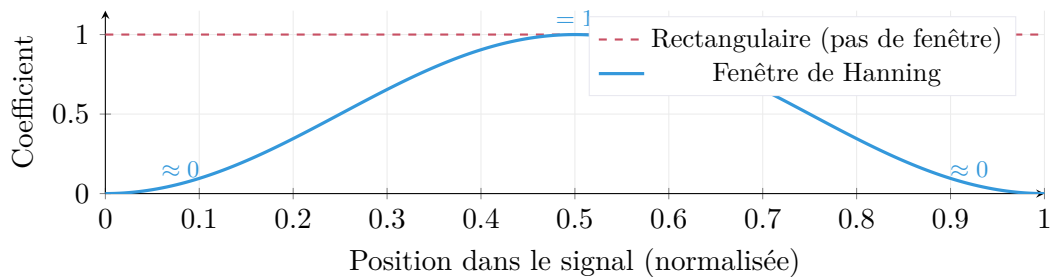
Figure 5 – La fenêtre de Hanning (bleu) atténue les bords vers 0, éliminant les discontinuités. Sans fenêtre (rouge pointillé), le signal garde sa pleine amplitude aux bords.
