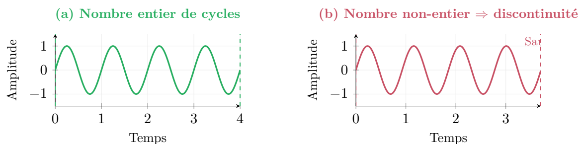
Figure 4 – (a) Si le signal contient un nombre entier de cycles, pas de discontinuité. (b) Sinon, un “saut” apparaît aux bords, créant de la fuite spectrale.
