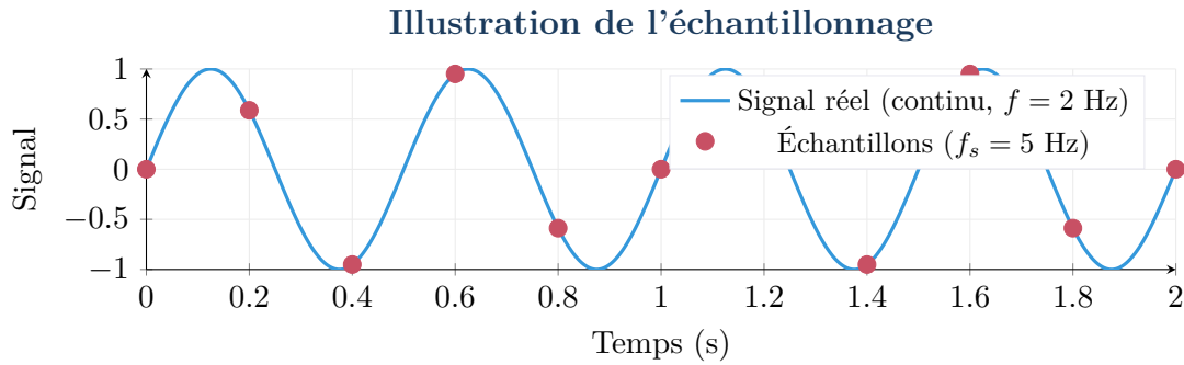
Figure 3 – Le signal continu (bleu) est mesuré uniquement aux points rouges. Avec f_s = 5 Hz et un signal à 2 Hz, on a 2.5 échantillons par cycle : suffisant (Nyquist respecté).
