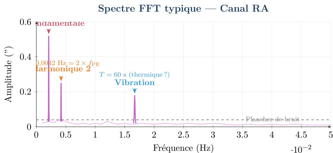
Figure 6 – Spectre FFT fictif mais réaliste montrant les éléments typiques à identifier
