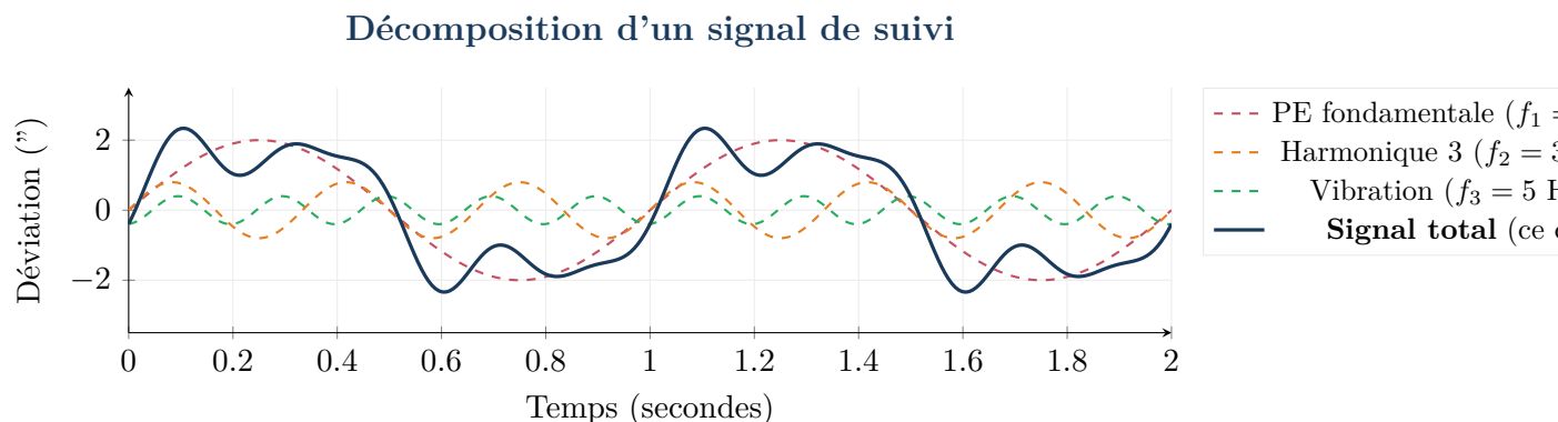
Figure 2 – Le signal bleu épais est la somme des trois composantes individuelles (tiretées). Fourier permet de retrouver chaque composante à partir du signal total.
