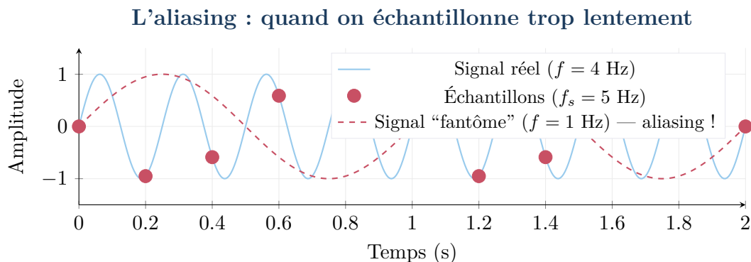
Figure 7 — Un signal à 4 Hz échantillonné à 5 Hz ( f_{\text{Nyquist}} = 2,5 \text{ Hz} ). La fréquence est au-dessus de Nyquist ! Les points d'échantillonnage (rouges) suggèrent un signal à 1 Hz (tiretés rouges) qui n'existe pas dans la réalité. C'est l' aliasing .
