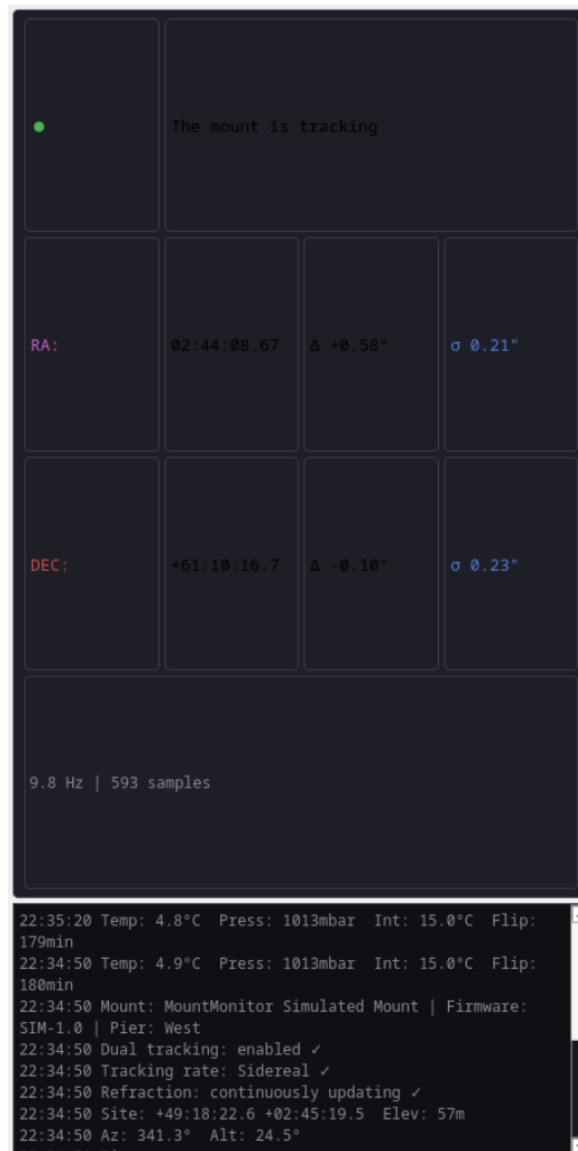
FIGURE 2.2 – Le bandeau d'état : voyant, coordonnées brutes, écart instantané, écart-type, cadence, puis le journal.
