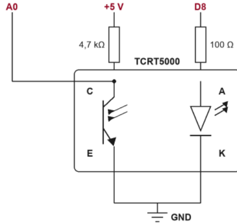
Figura 1: Ligação do TCRT5000 ao Arduino Mega.
