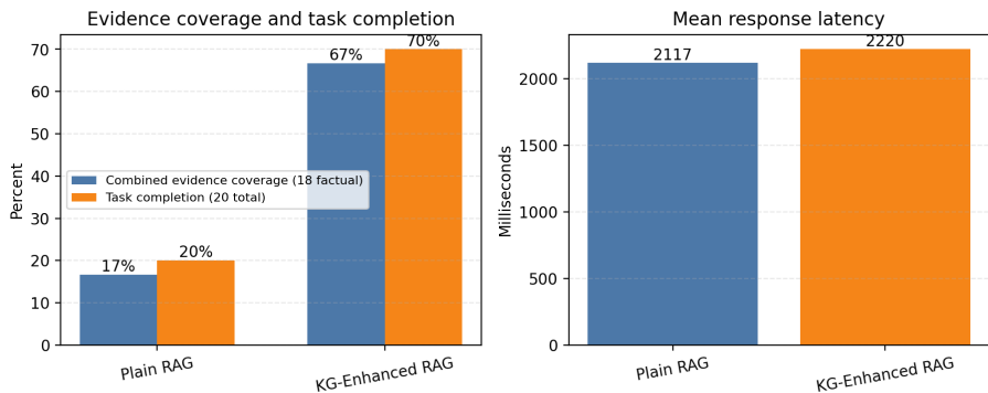
图 5-7 答案要点证据覆盖率、任务完成率与响应时延
