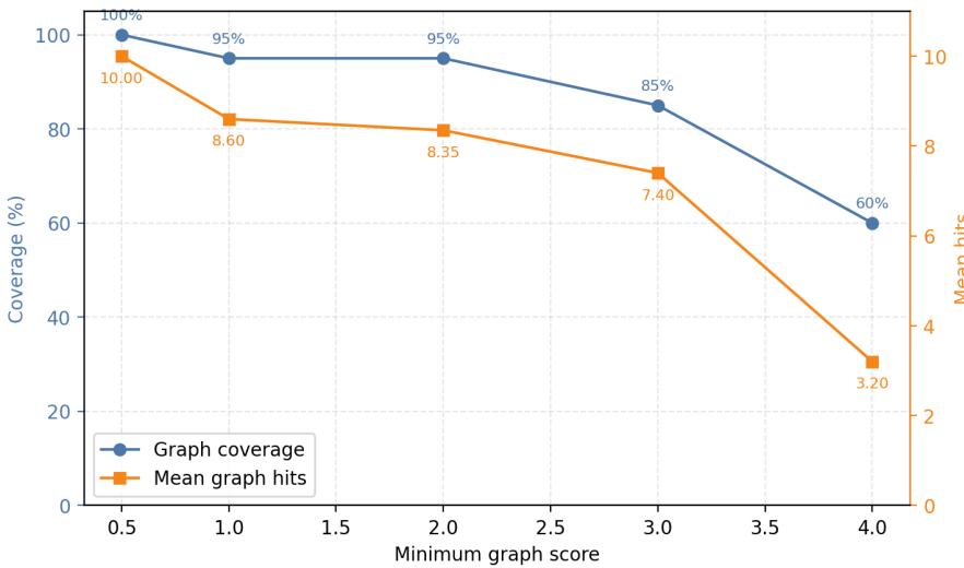
图 5-8 图谱最低得分阈值敏感性
