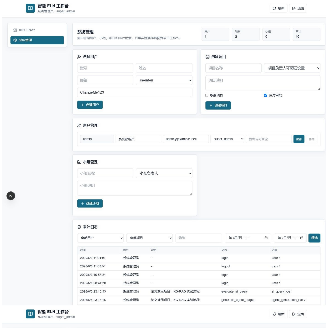
图 6-3 系统用户与全局角色管理界面
