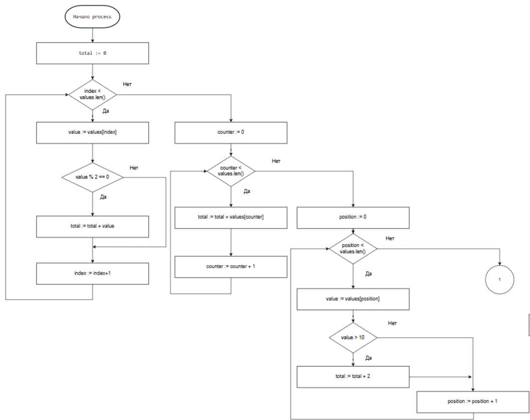
Рисунок 3 – Схема алгоритма программы, часть 1(функция process)
