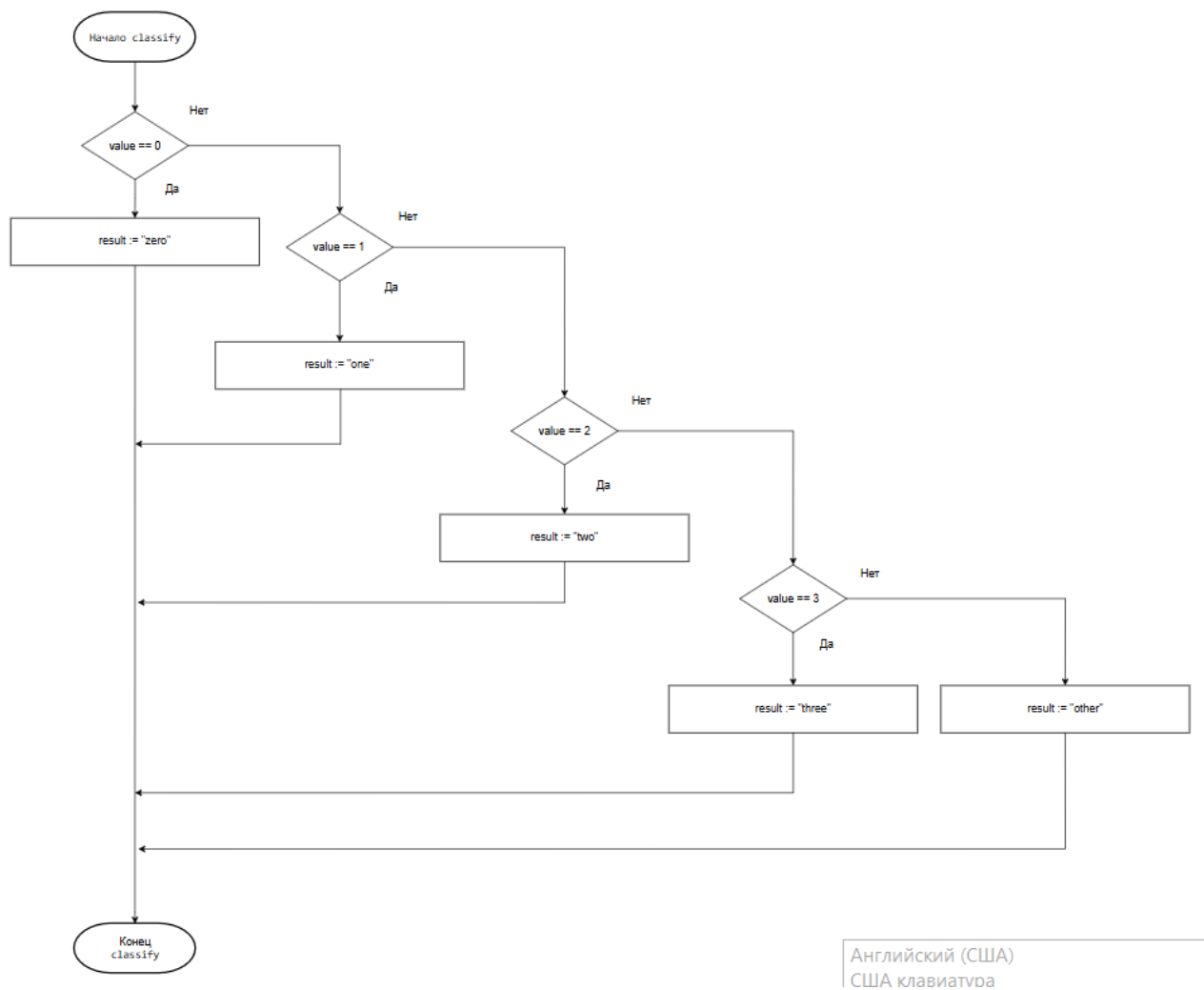
Рисунок 2 – Схема алгоритма программы (функция classify )
