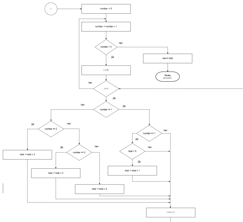
Рисунок 4 – Схема алгоритма программы, часть 2 (функция process)
