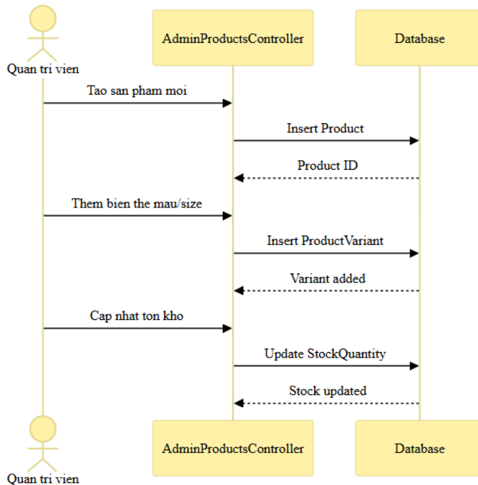
Hình 3.2: Luồng tuần tự quản trị biến thể sản phẩm
