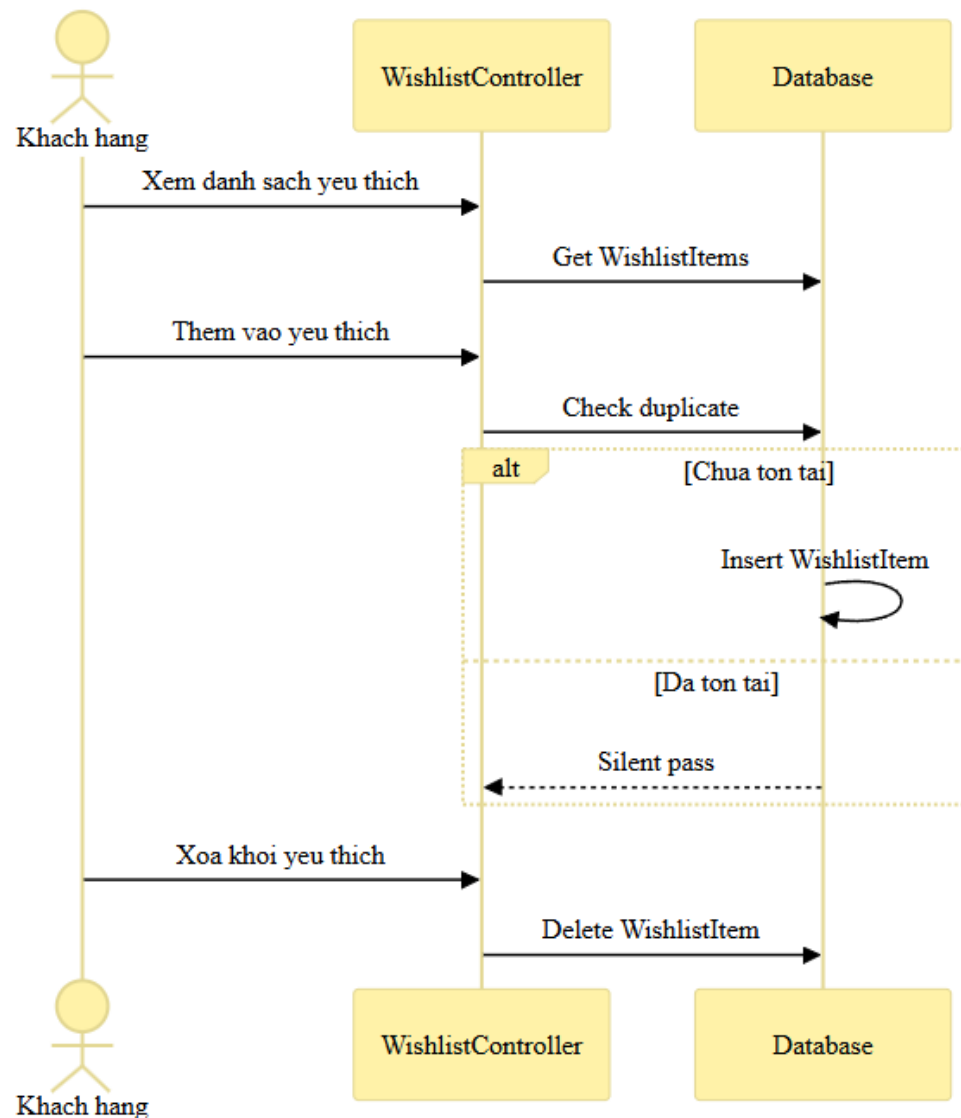
Hình 3.4: Luồng tuần tự khách hàng quản lý wishlist
