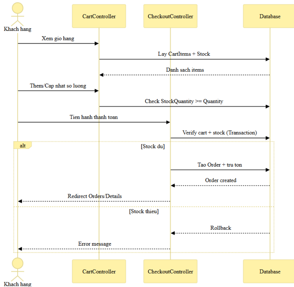
Hình 3.3: Luồng tuần tự khách hàng checkout
