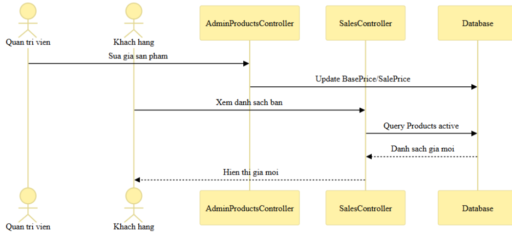
Hình 3.5: Luồng tuần tự cập nhật giá
