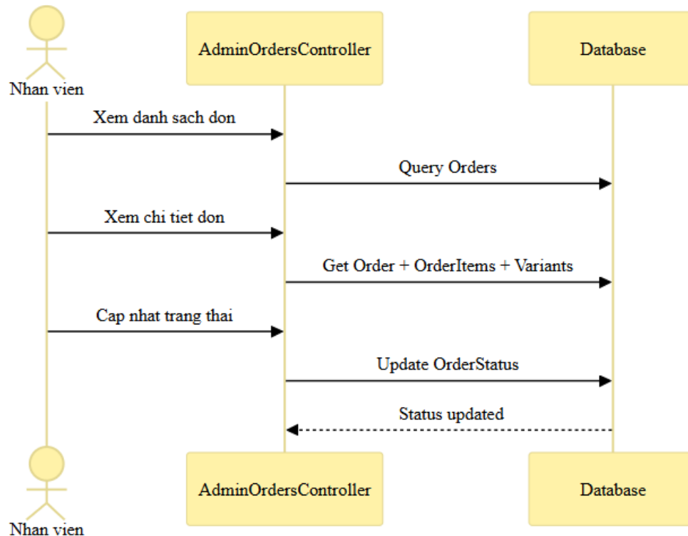
Hình 3.6: Luồng tuần tự nhân viên xử lý đơn hàng
