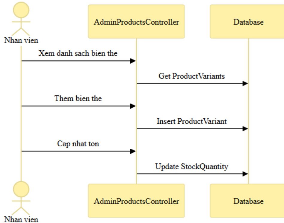
Hình 3.7: Luồng tuần tự quản lý tồn kho biến thể
