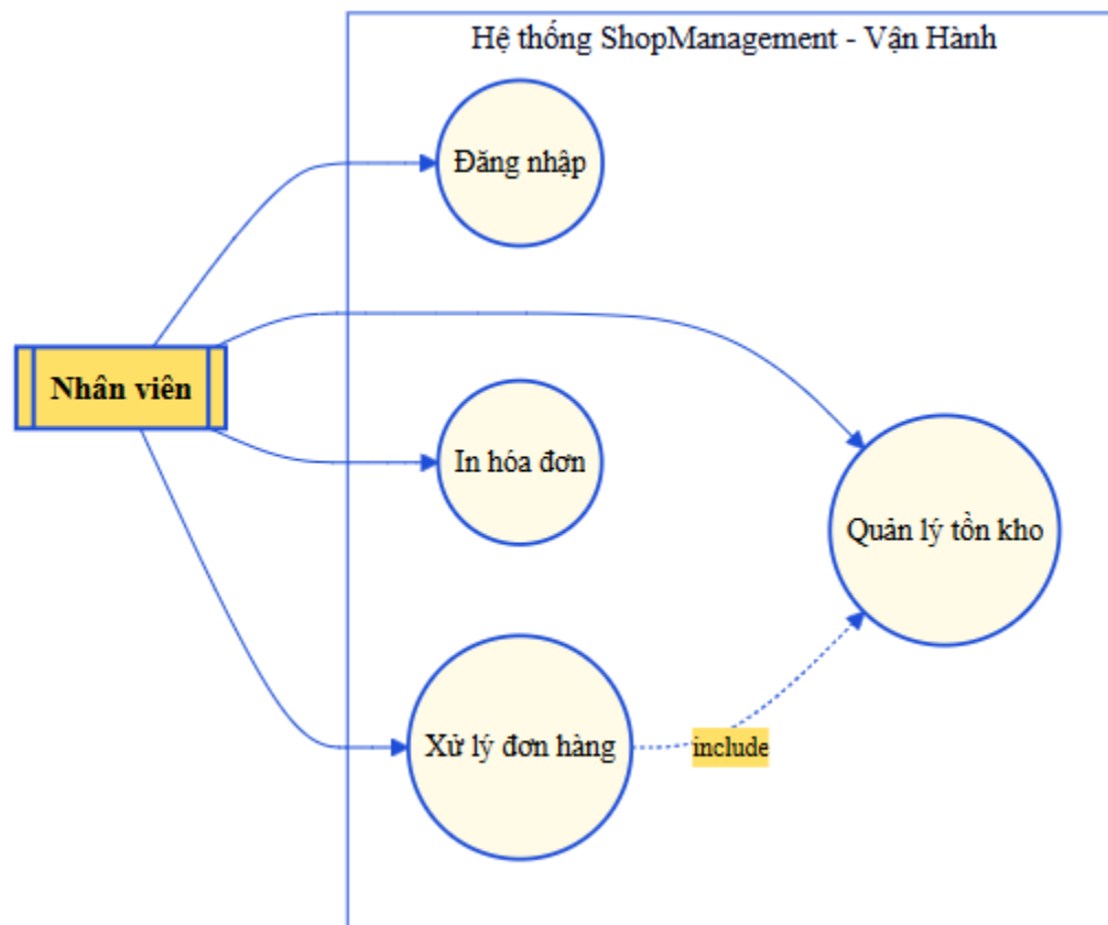
Hình : Use case tổng quát chức năng nhân viên bán hàng
