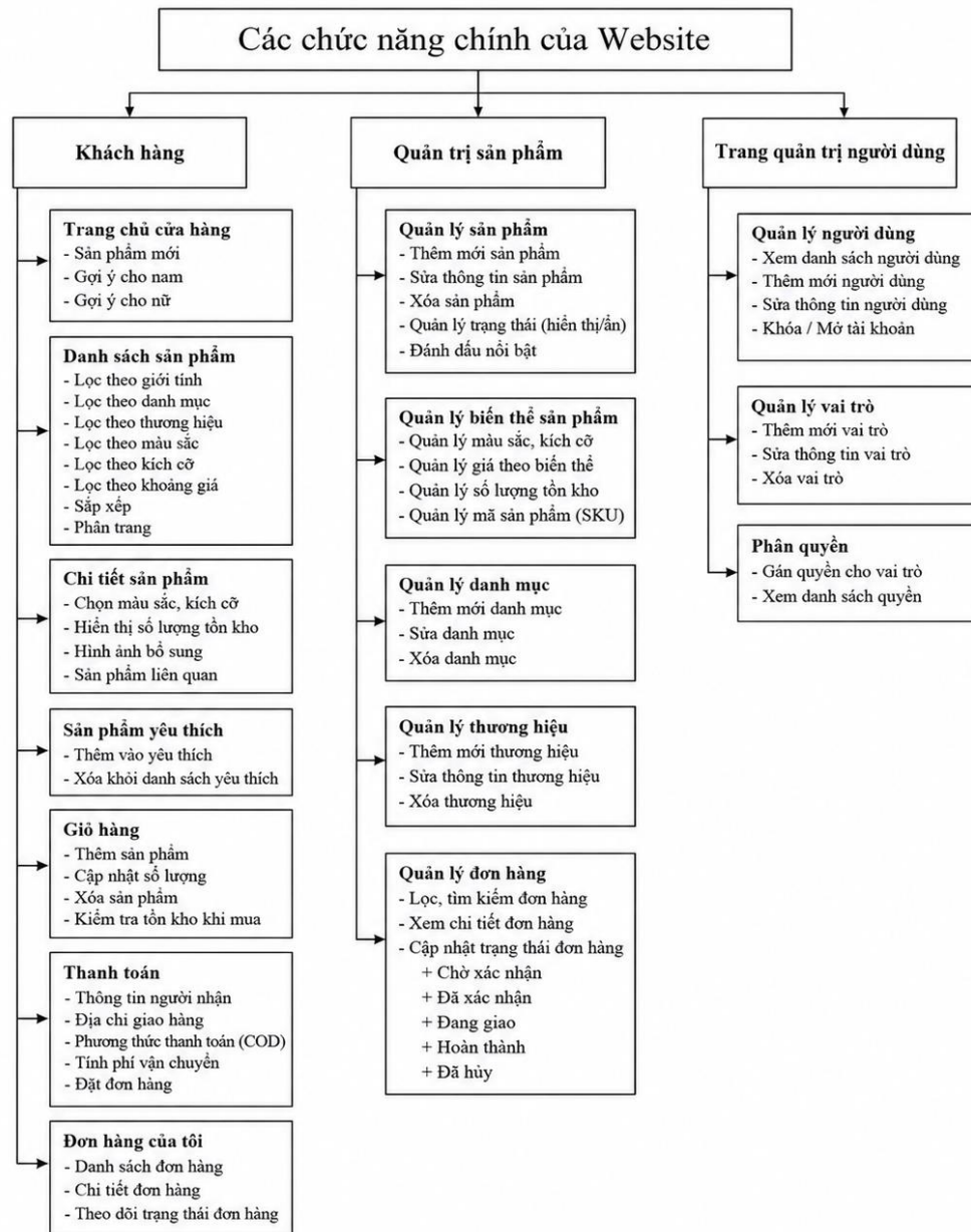
Hình: Sơ đồ chức năng
