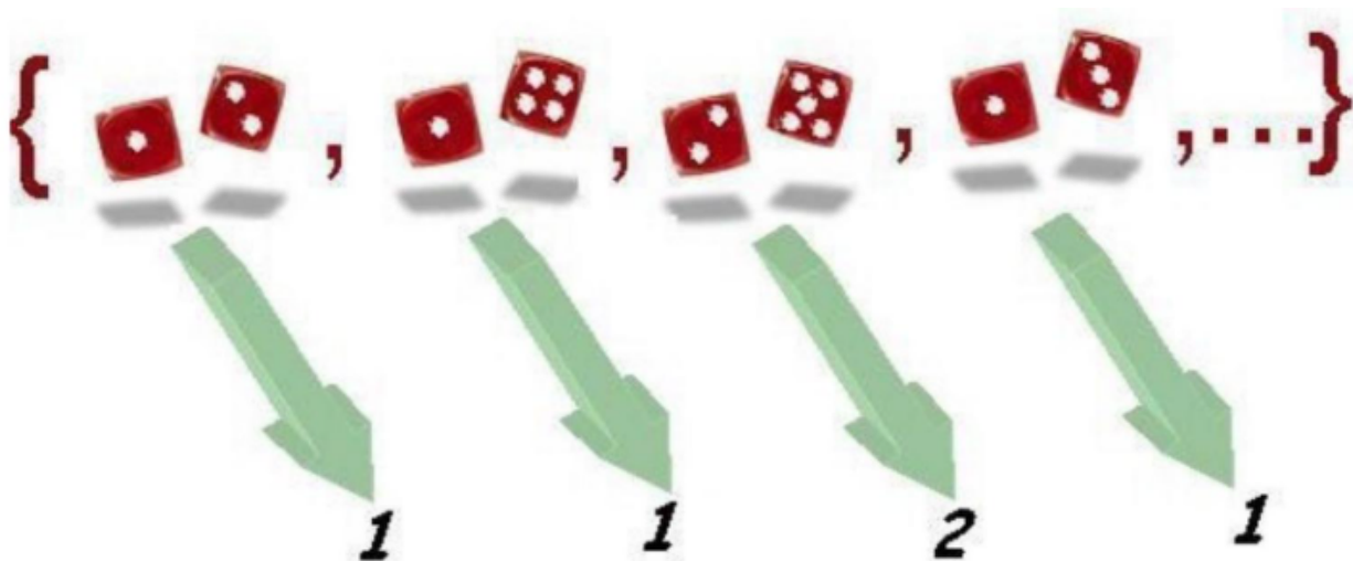
Figure 7: Asignación del mínimo de las caras.
