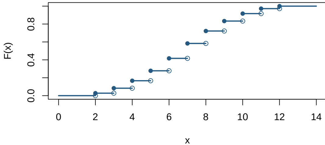
Figure 2: CDF de la suma de dos dados: continua por la derecha.
