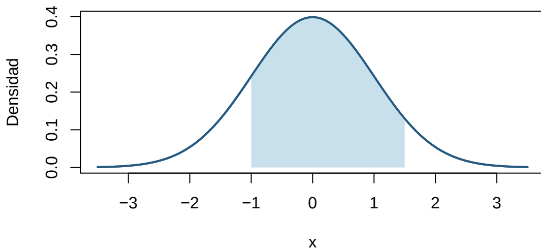
Figure 4: Probabilidad como área bajo una densidad normal estándar; distinta del ejemplo de estaturas.
