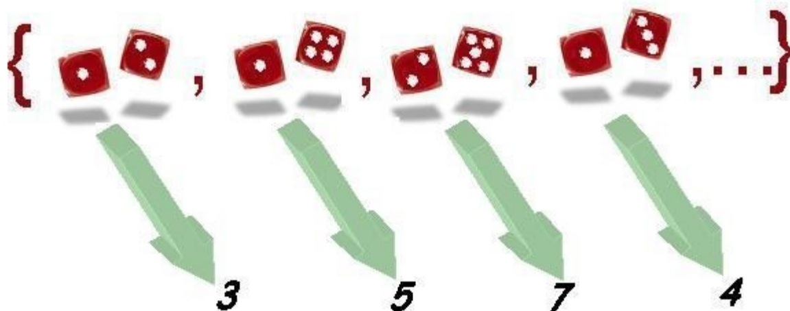
Figure 6: Asignación de la suma de puntos.
