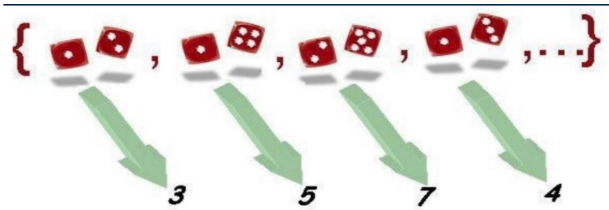
Figure 8: Variable suma de dos dados.
