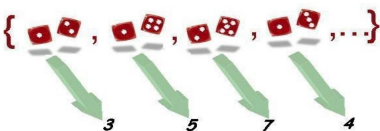
Figure 11: Suma de puntos y valores posibles.
