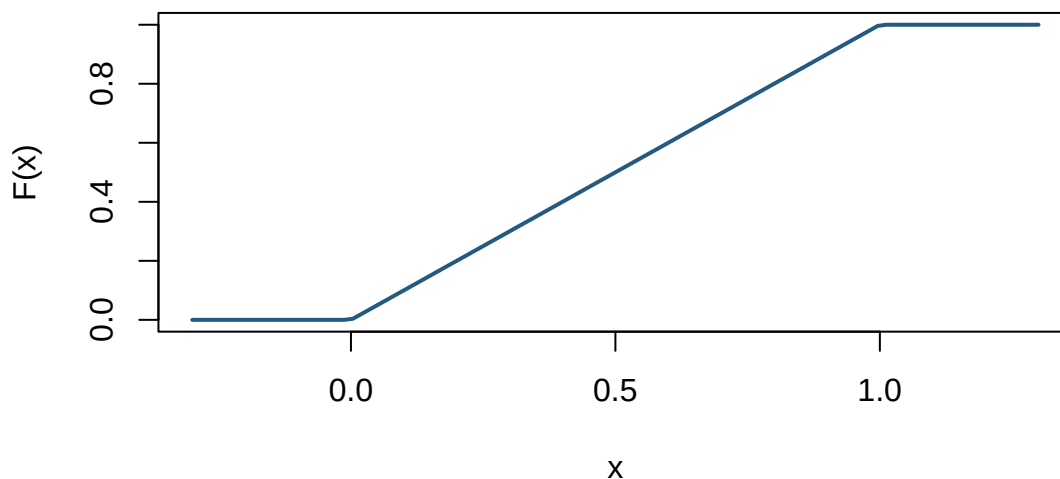
Figure 1: Función de distribución continua de una uniforme en (0,1) .
