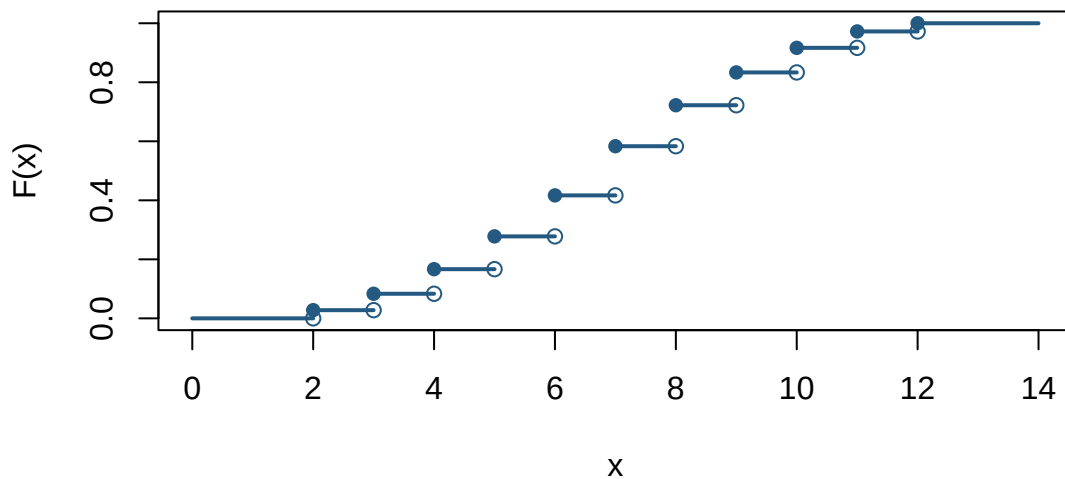
Figure 10: CDF de la suma de dos dados regulares e independientes.
