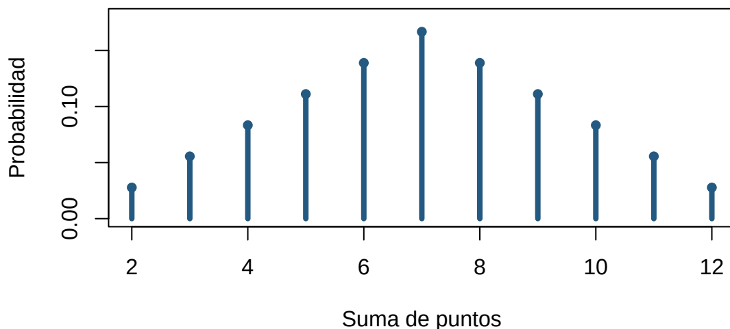
Figure 12: Masa de probabilidad de la suma de dos dados.
