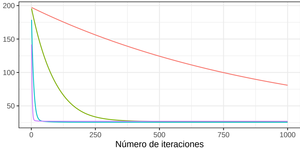
Evolución del error en validación cruzada vs tasa de aprendizaje
