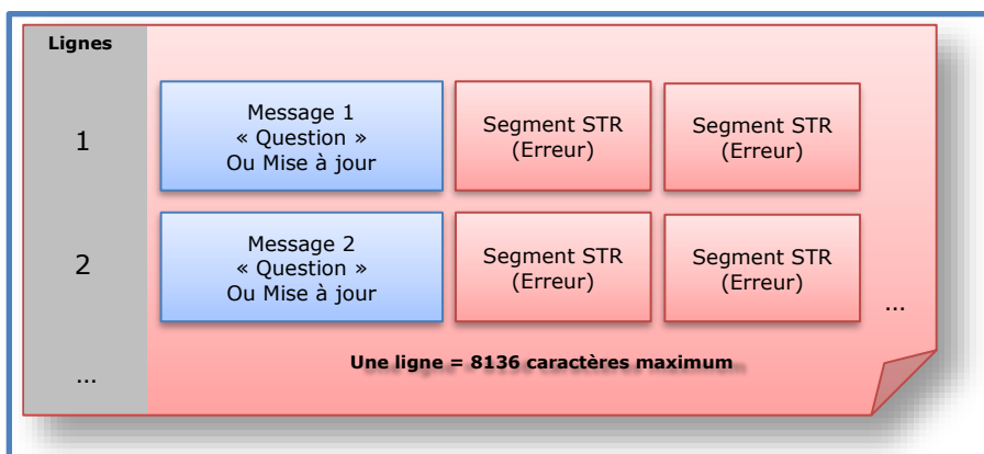
Fig. 4 - Structure d'un fichier "Réponse" avec rejet
