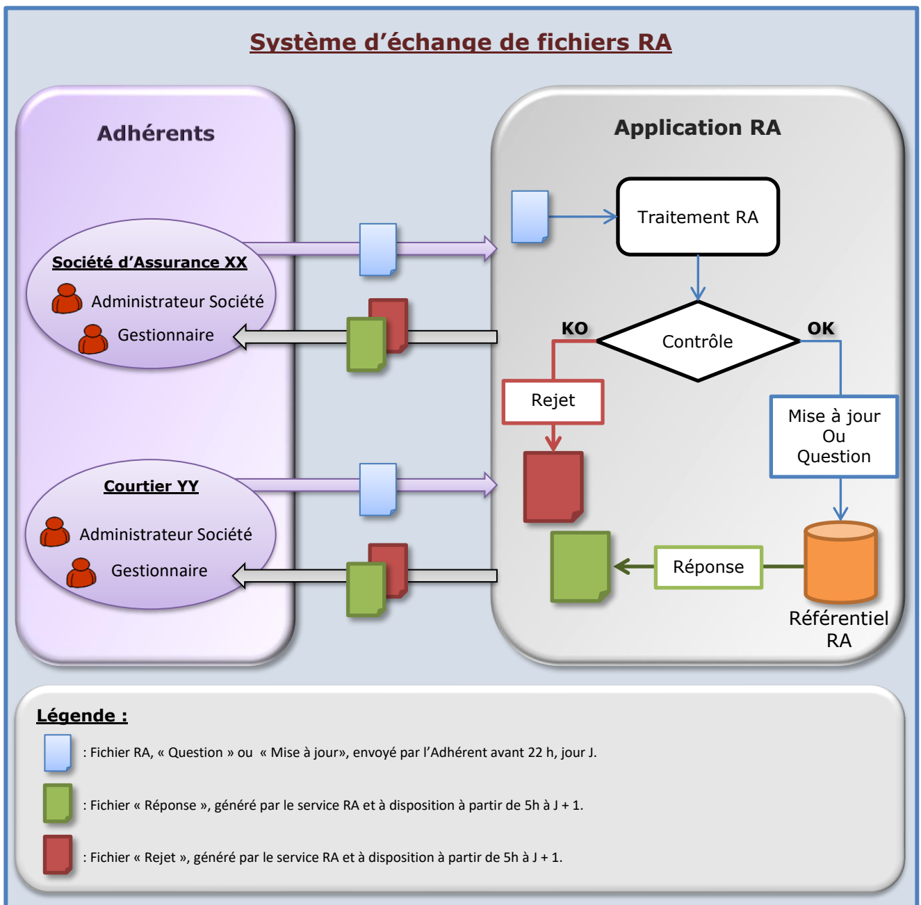
Fig. 2 - Descriptif des échanges de fichiers RA
