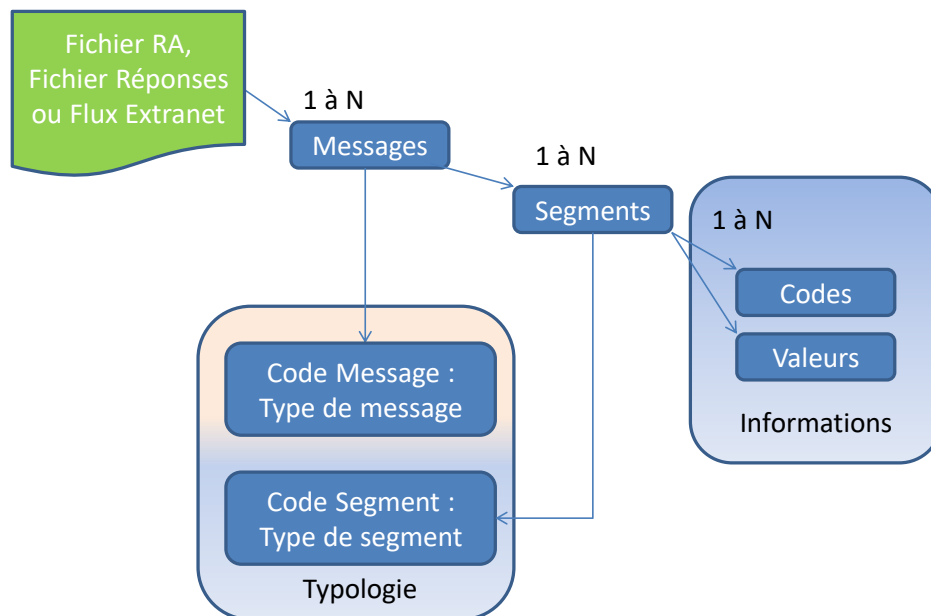
Fig. 1 - Structure d'un message
