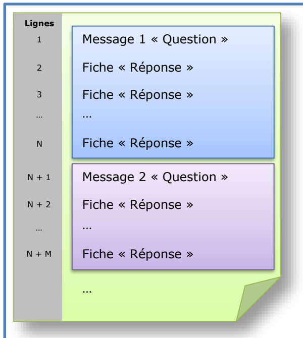
Fig. 3 - Structure d'un fichier "Réponse"
